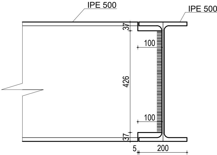
Detaj D1
