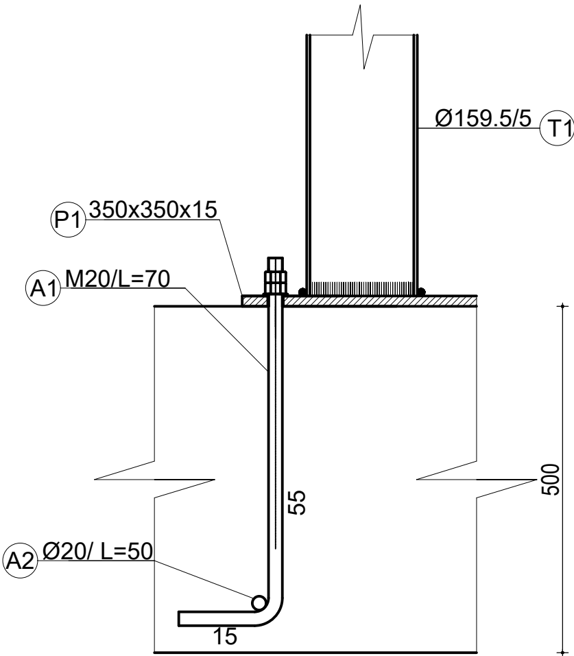
DETAJ I BASHKIMIT TE KOLONES METALIKE ME THEMELIN
