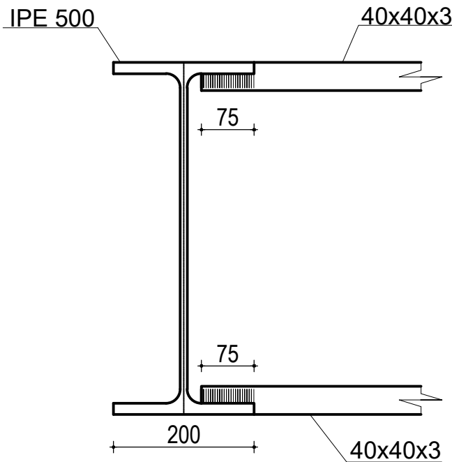
DETAJ I BASHKIMIT TE PROFILIT IPE 500 ME PROFILIN 40X40X3
