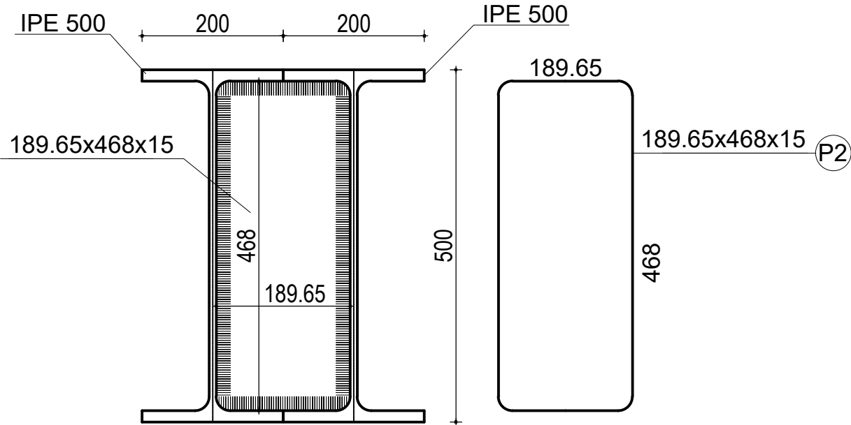
Detaj D2
