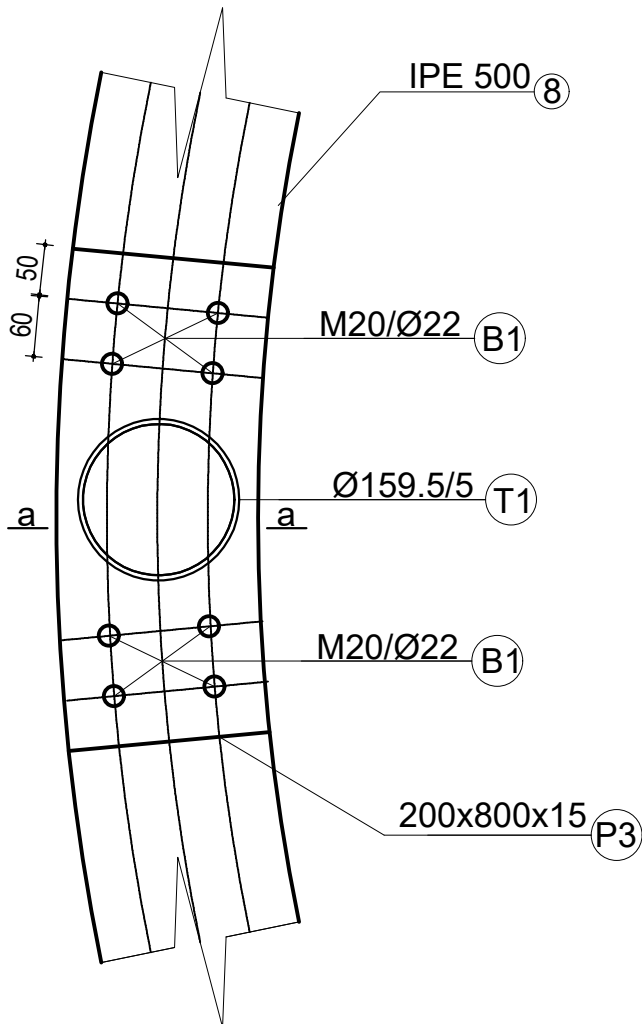
DETAJ I BASHKIMIT TE KOLONES METALIKE ME PROFILIN IPE 500
