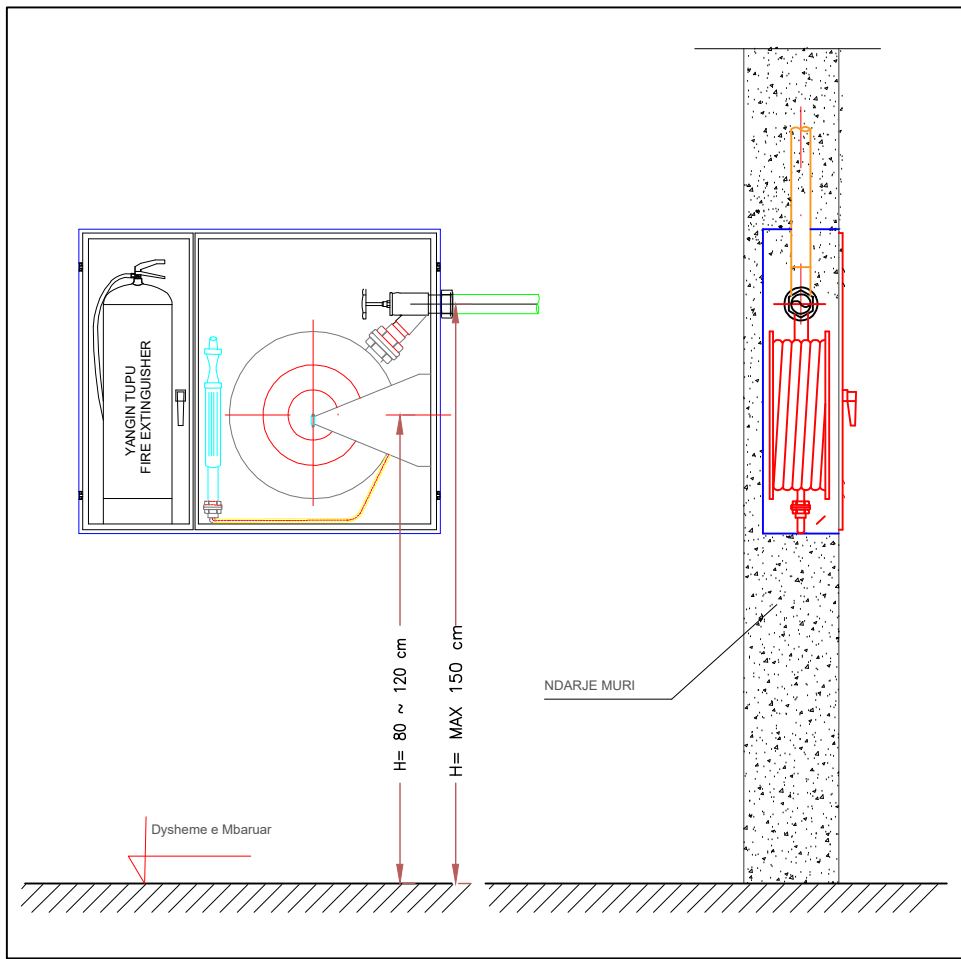
Detaji i Vendosijes se Hidrantit dhe Fikeses Portabel - E inkasuar ne mur, kapak metalik
