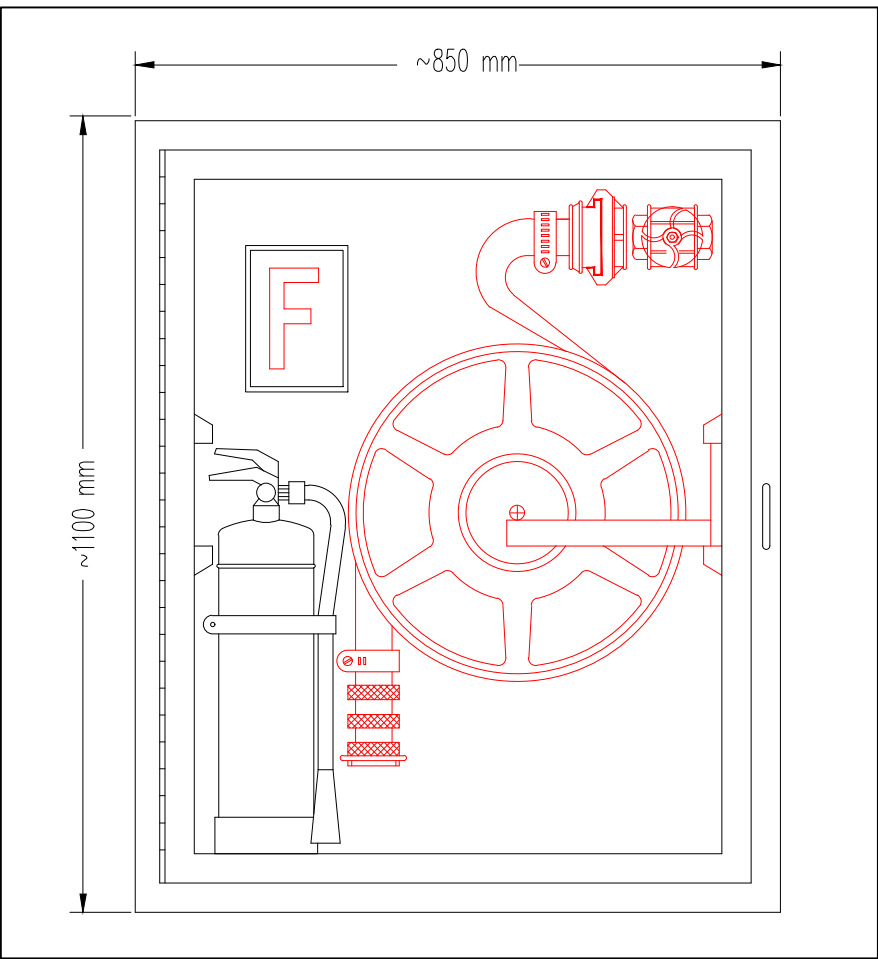
Permasat e Kutise se Hidrantit - E inkasuar ne mur, kapak metalik
