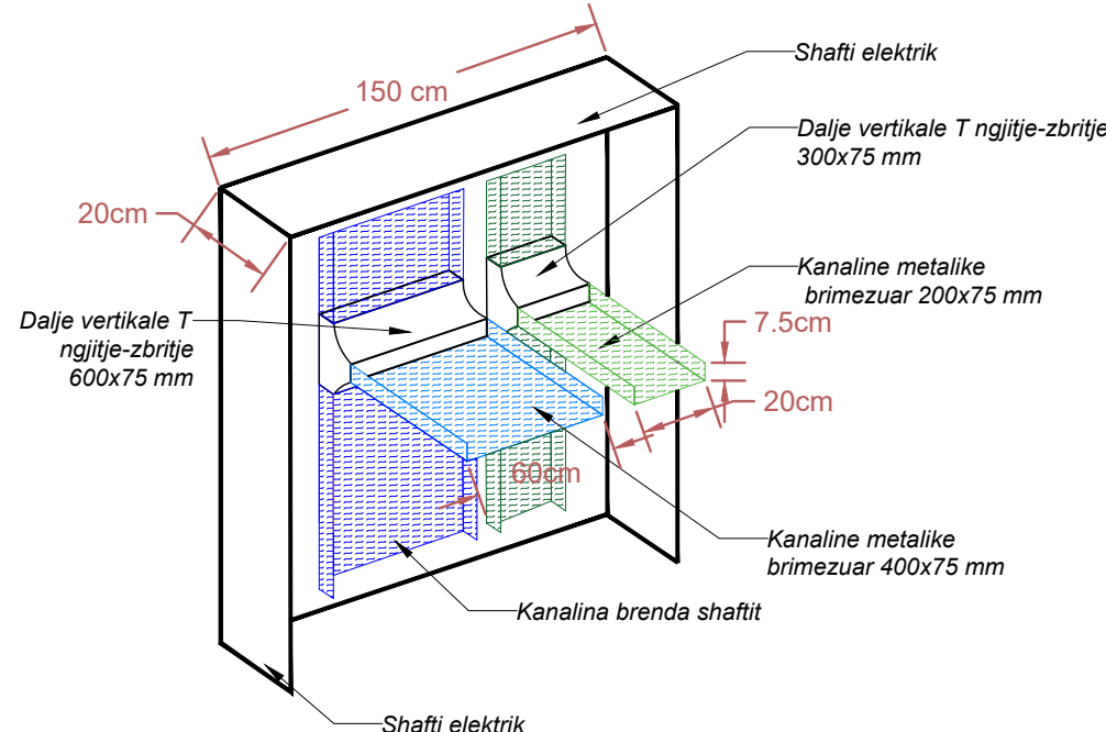
DETAJ 1 Ngjitja-Zbritja ne shaft
