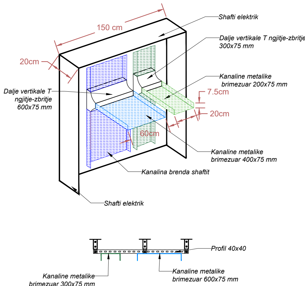
DETAJ 1 Ngjitja-Zbritja ne shaft
