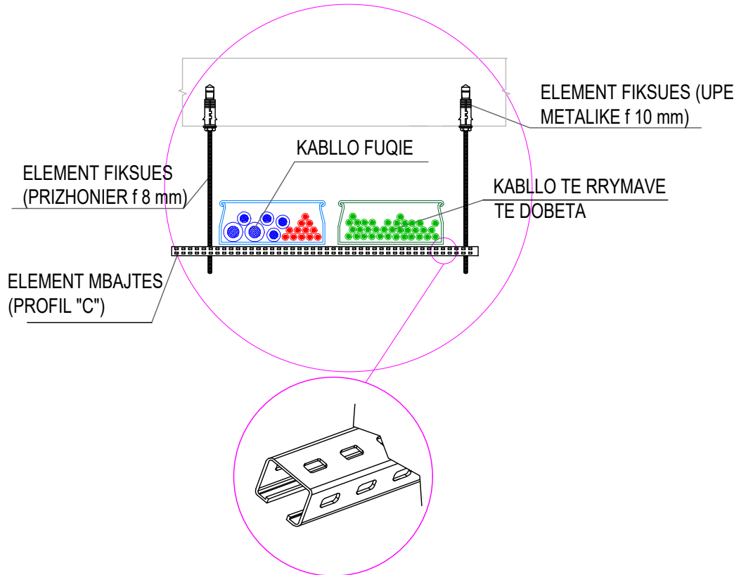
DETAJ I KANALINES METALIKE
