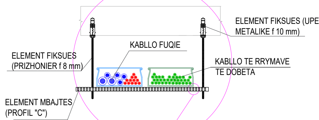
DETAJ I KANALINES METALIKE
