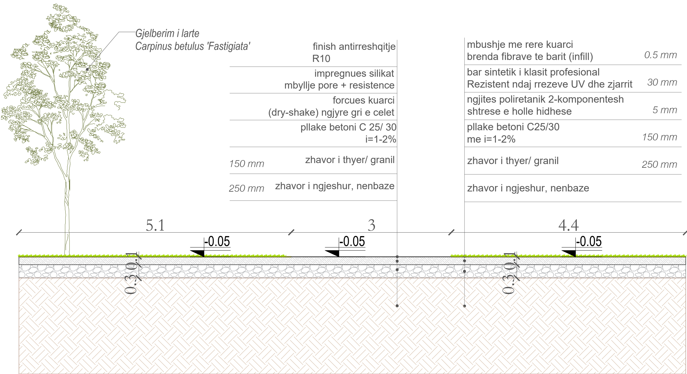
D1 - PRERJA 1 - 1 ; SH. 1:3
