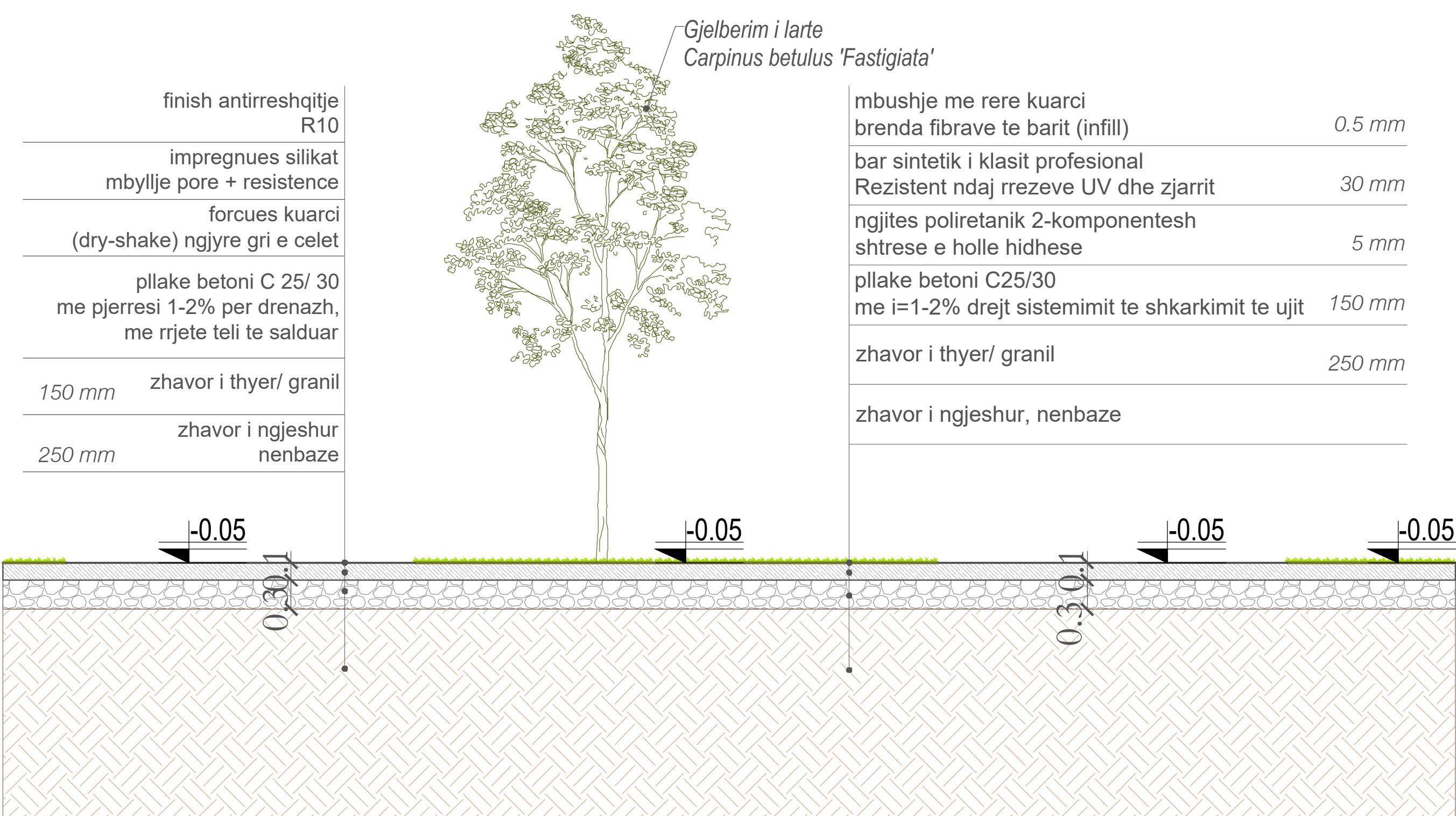
D2 - PRERJA 2 - 2 ; SH. 1:3
