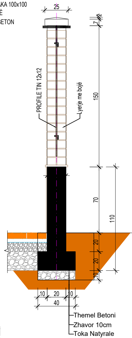
PRERJE B-B, Sh.1:25
