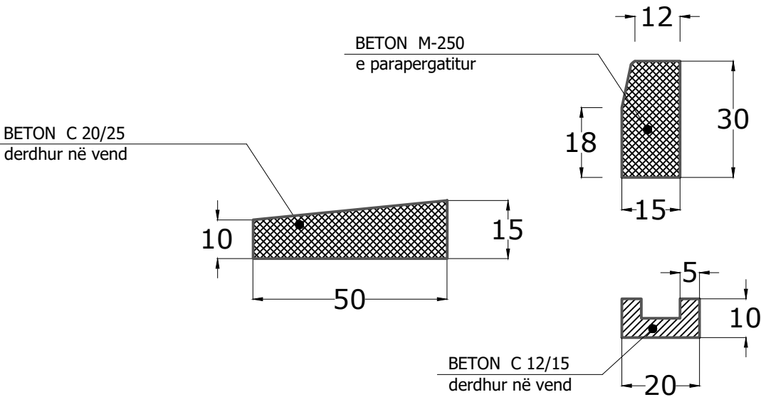
Detaji i Bordurës dhe kunetes Sh 1:15
