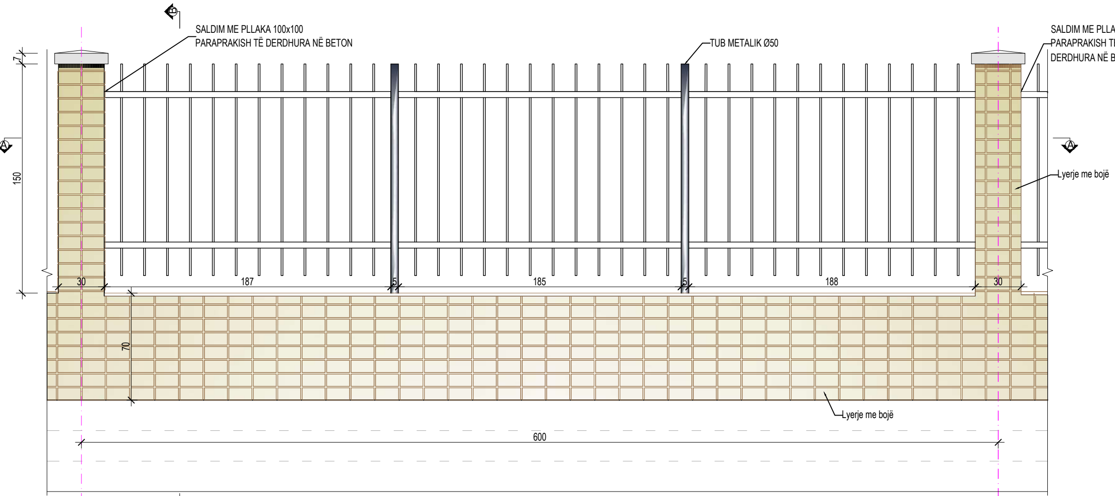
PAMJE NGA LART, Sh.1:25
