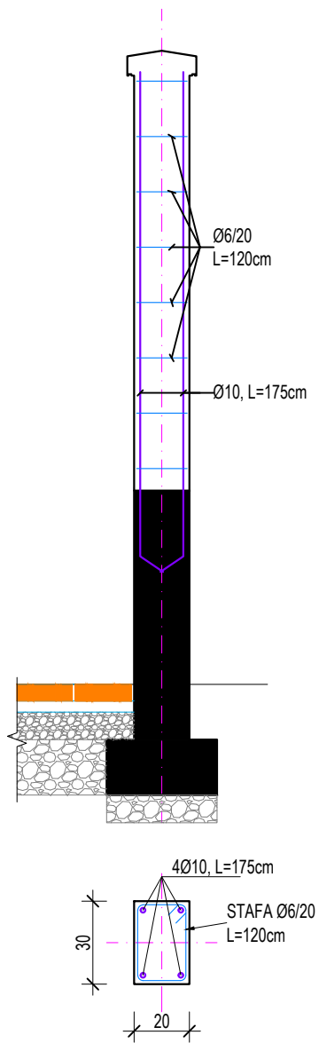
ARMIMI I KOLLONETËS, Sh.1:25
