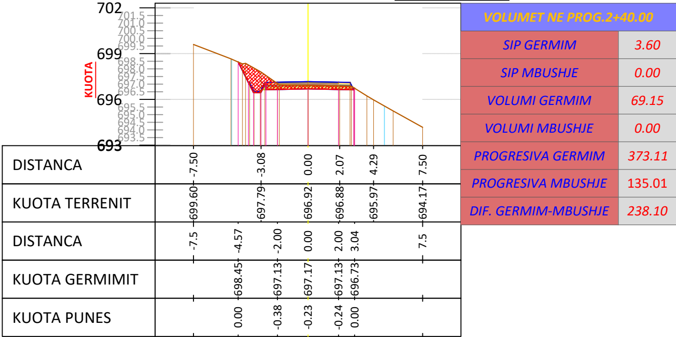
SC - 13 PROGRESIV. 0+240 m
