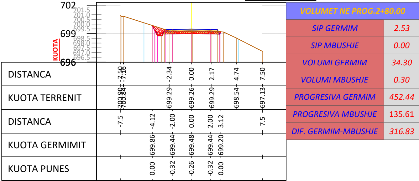
SC - 15 PROGRESIV. 0+280 m
