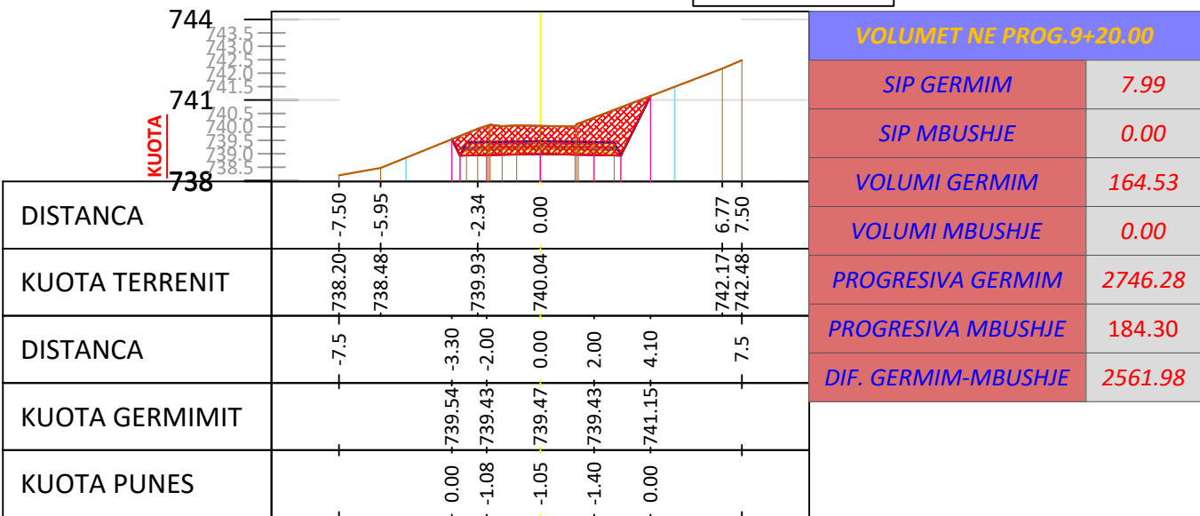
SC - 47 PROGRESIV. 0+920 m
