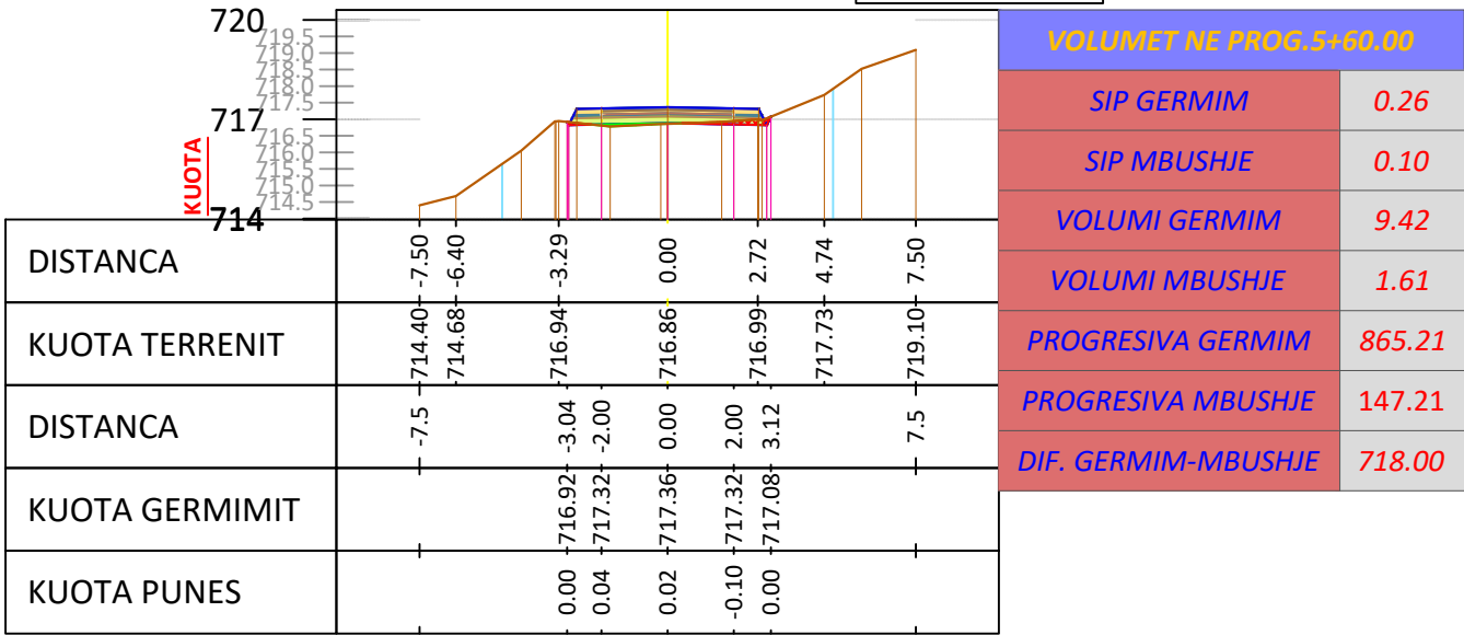
SC - 29 PROGRESIV. 0+560 m
