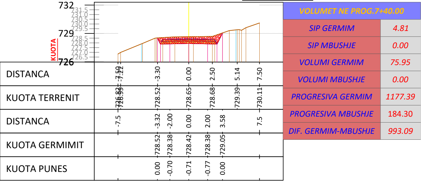
SC - 38 PROGRESIV. 0+740 m
