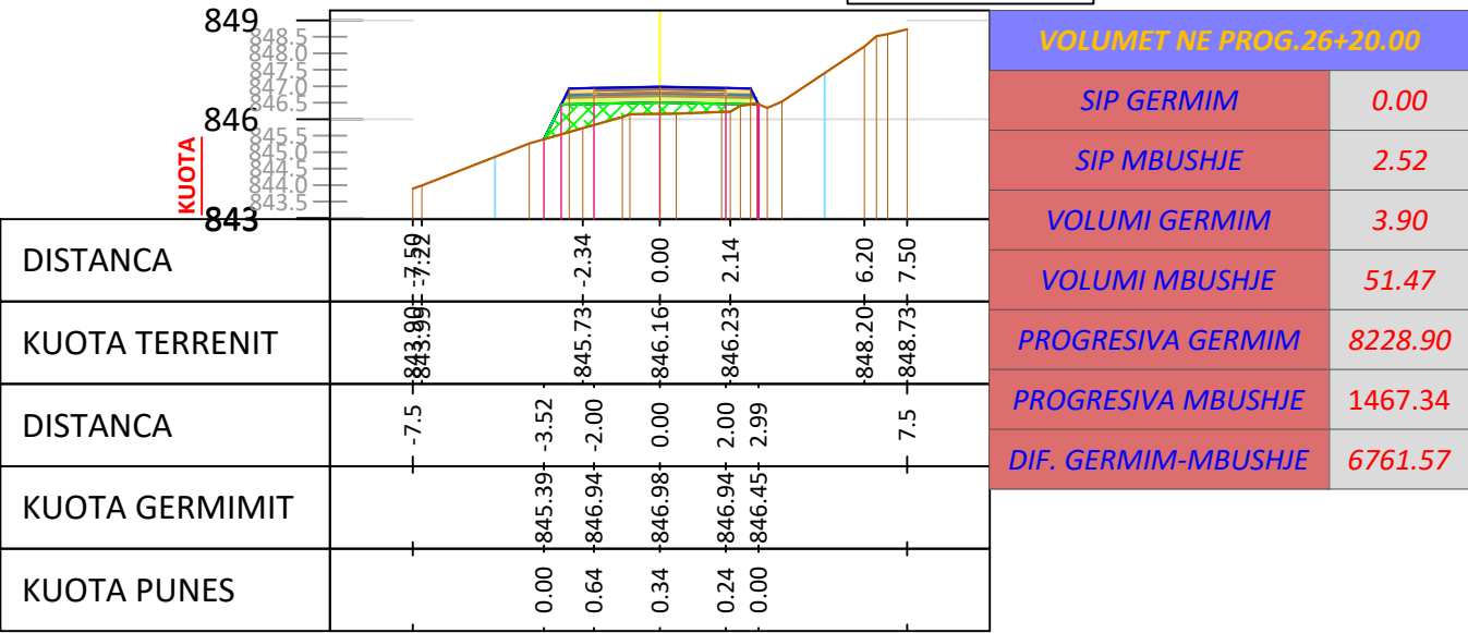
SC - 132 PROGRESIV. 2+620 m
