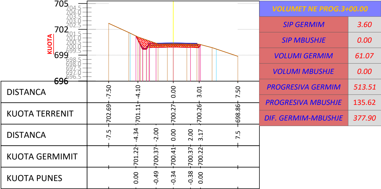
SC - 16 PROGRESIV. 0+300 m
