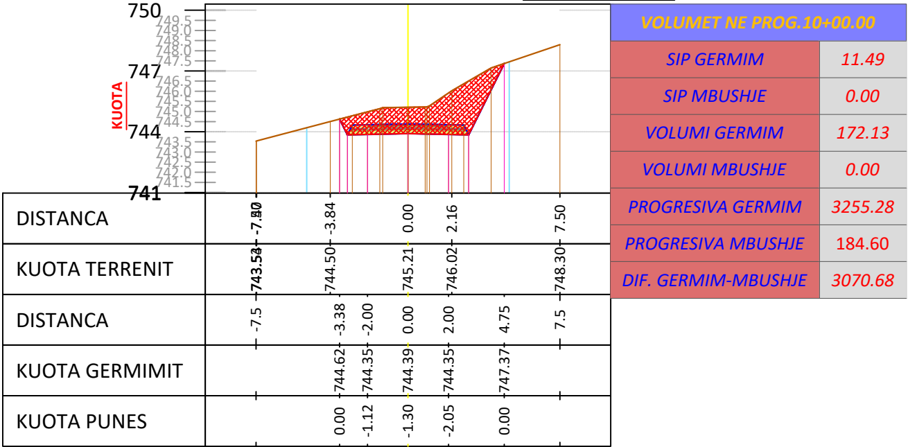
SC - 51 PROGRESIV. 1+000 m
