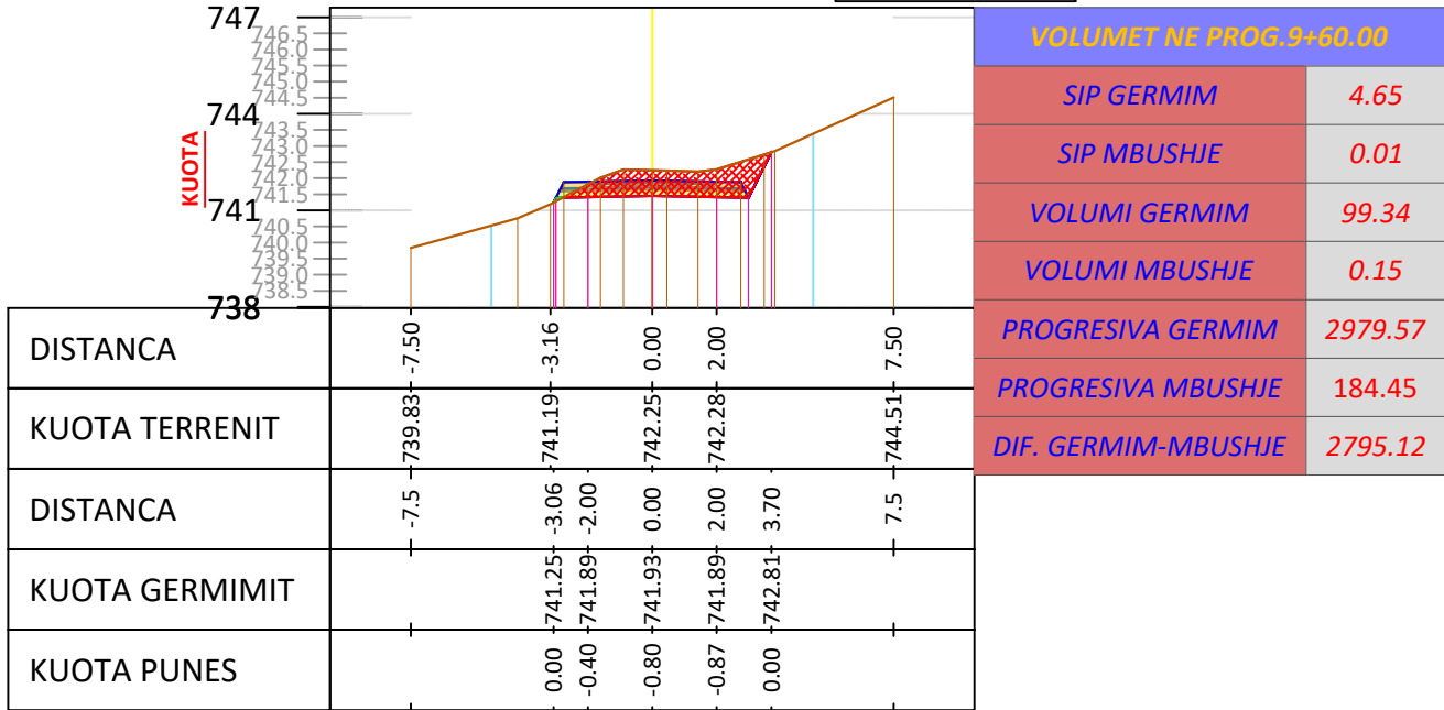
SC - 49 PROGRESIV. 0+960 m
