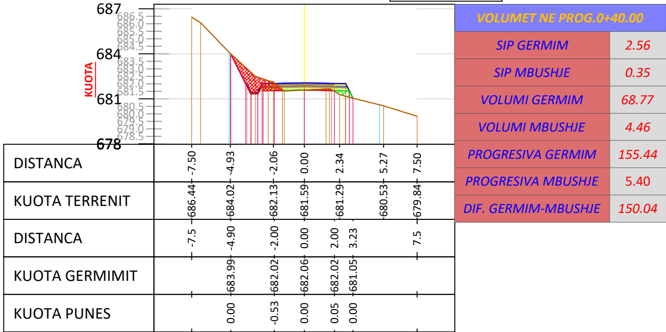
SC - 3 PROGRESIV. 0+040 m
