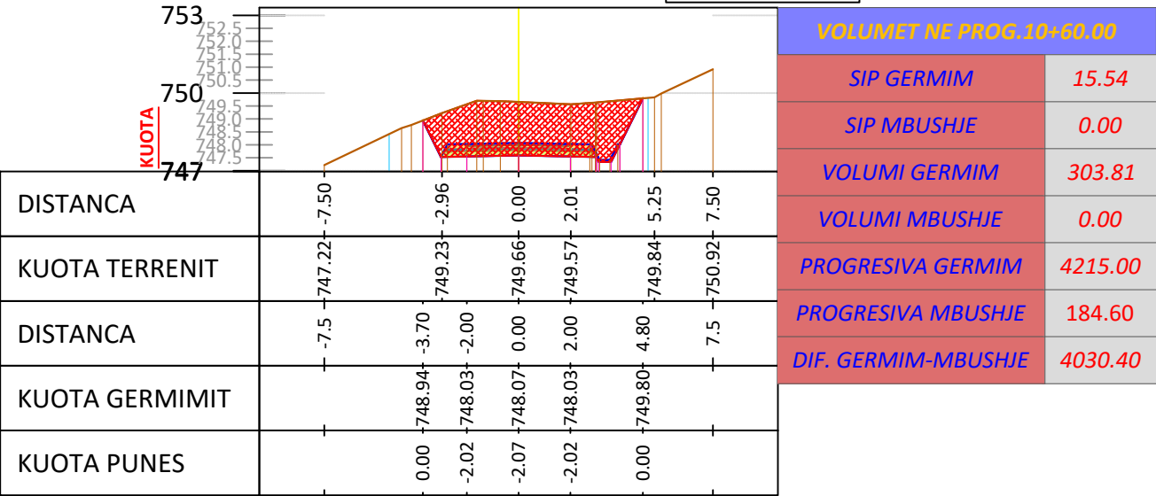
SC - 54 PROGRESIV. 1+060 m
