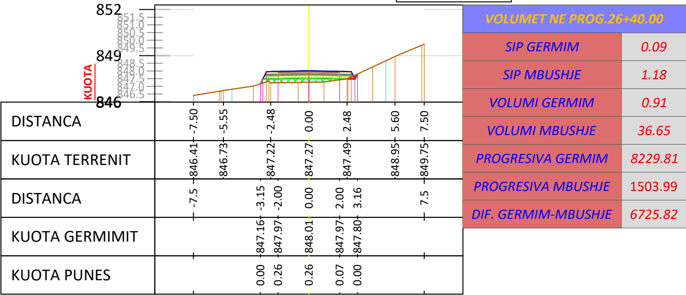
SC - 133 PROGRESIV. 2+640 m
