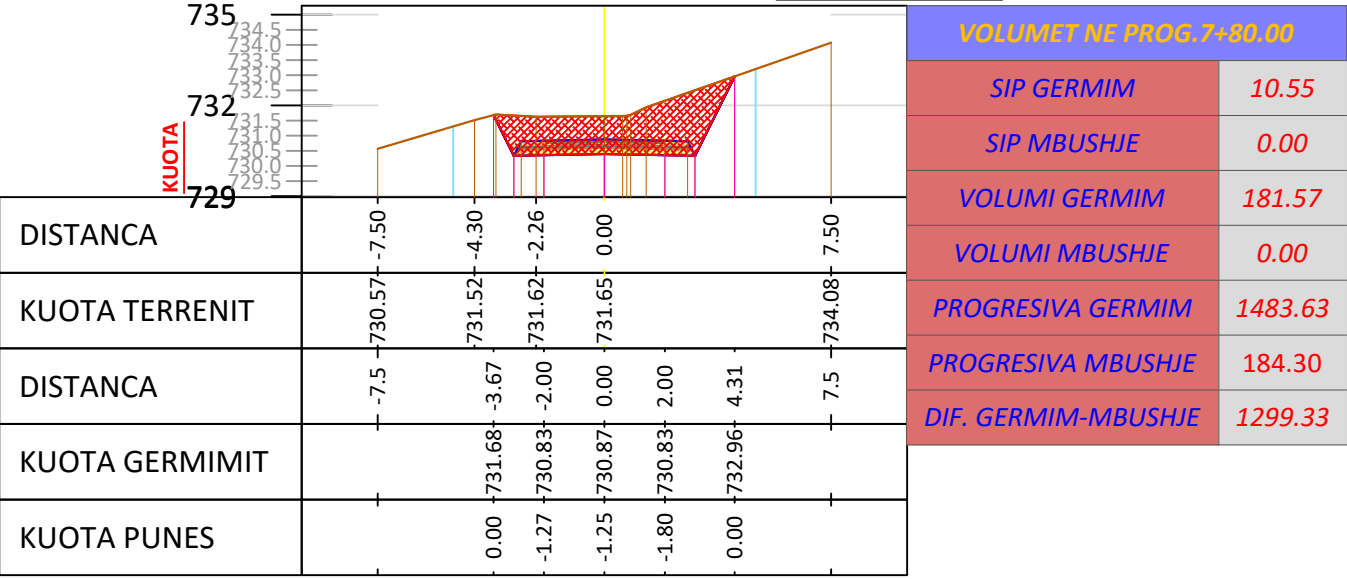
SC - 40 PROGRESIV. 0+780 m
