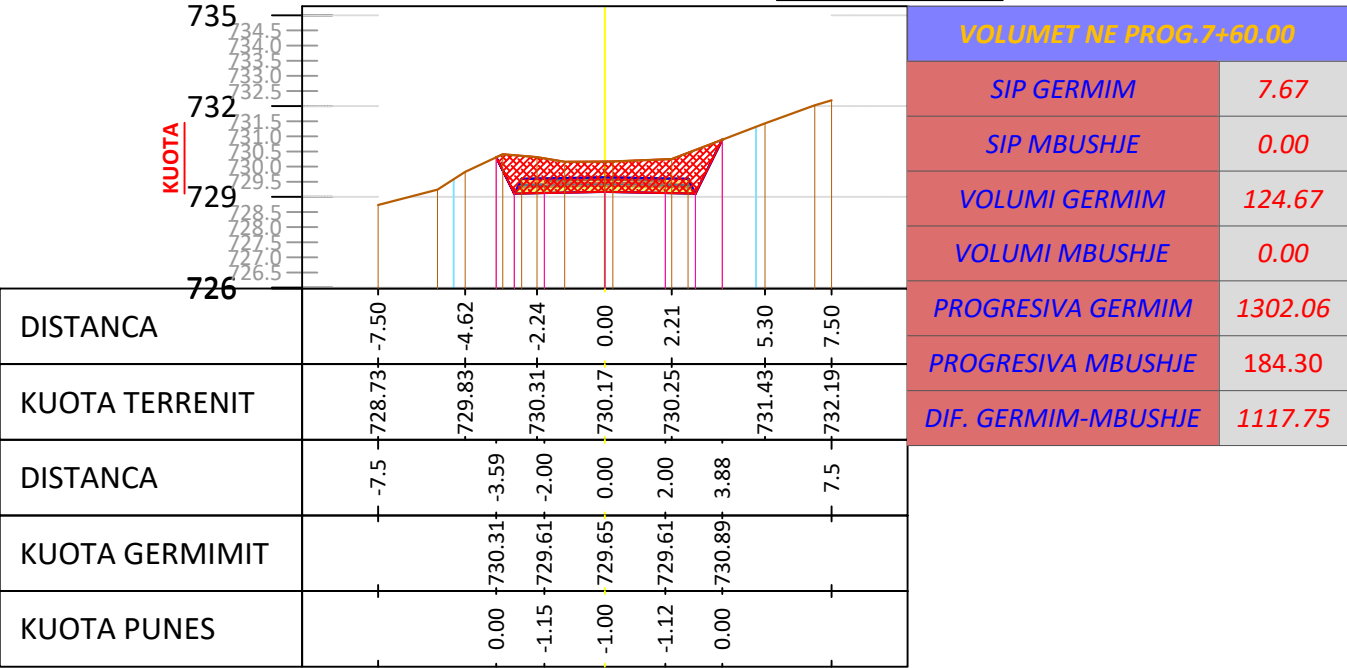
SC - 39 PROGRESIV. 0+760 m
