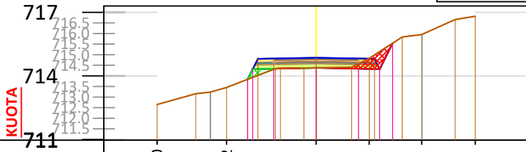
SC - 27 PROGRESIV. 0+520 m
