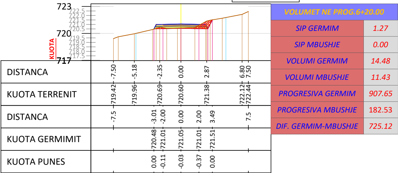
SC - 32 PROGRESIV. 0+620 m
