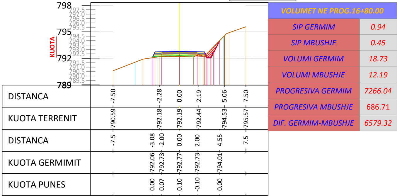
SC - 85 PROGRESIV. 1+680 m
