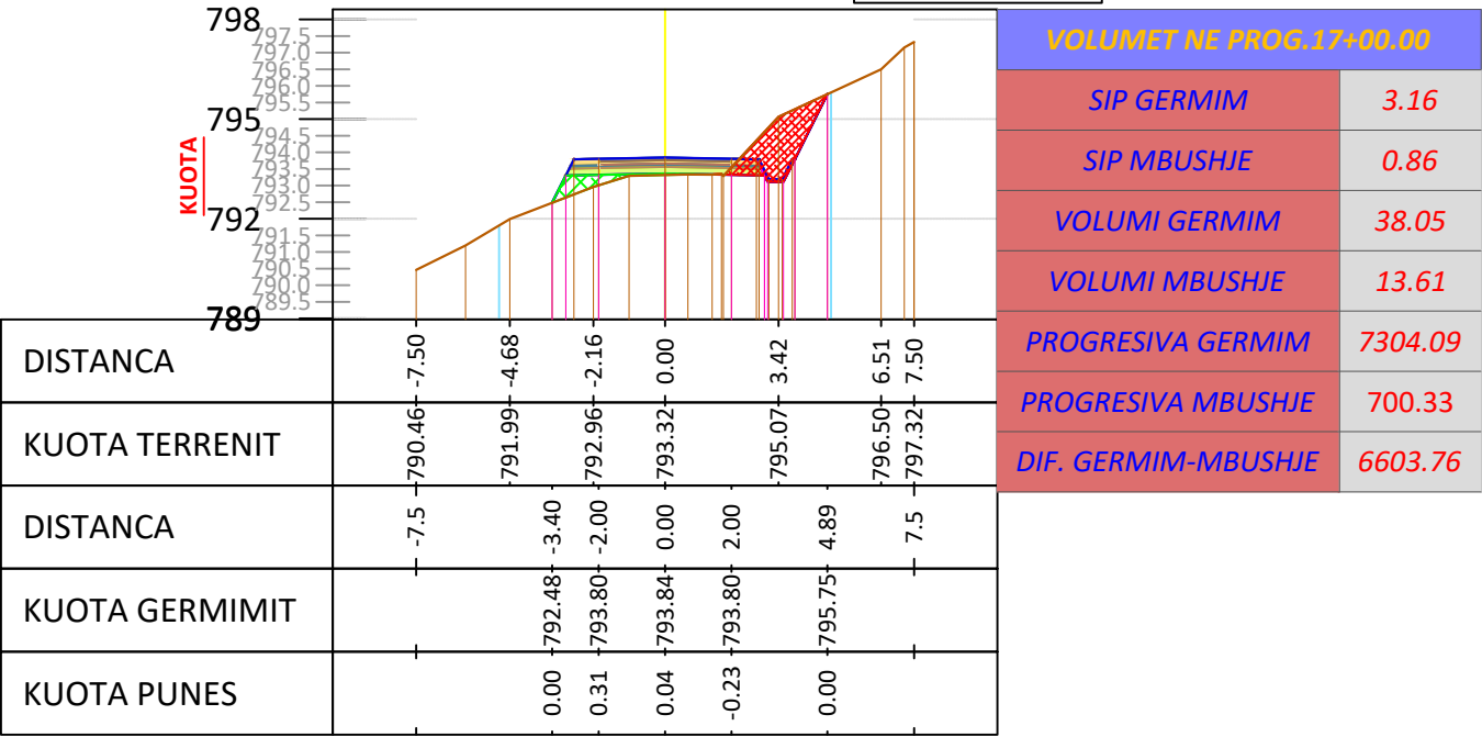
SC - 86 PROGRESIV. 1+700 m
