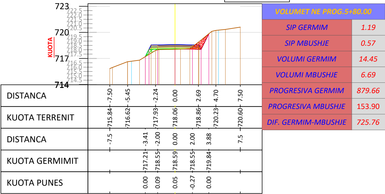
SC - 30 PROGRESIV. 0+580 m
