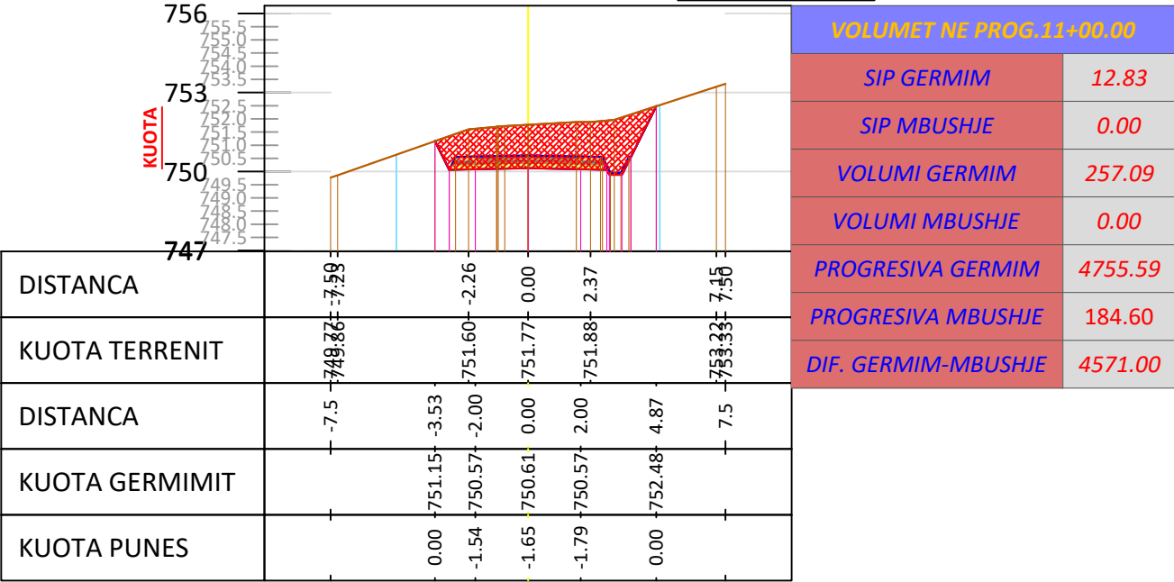
SC - 56 PROGRESIV. 1+100 m
