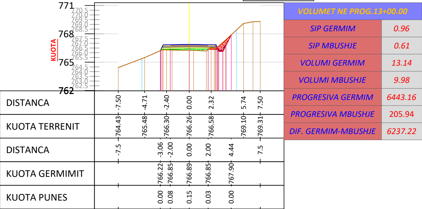
SC - 66 PROGRESIV. 1+300 m
