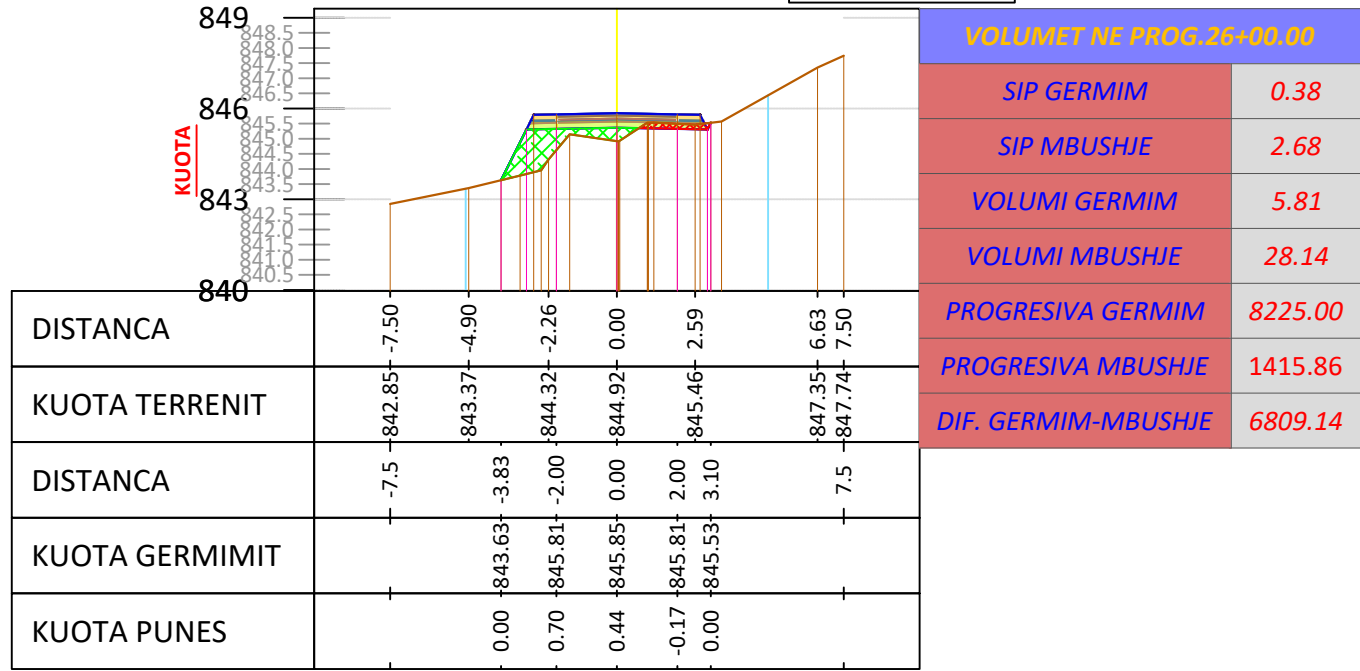
SC - 131 PROGRESIV. 2+600 m
