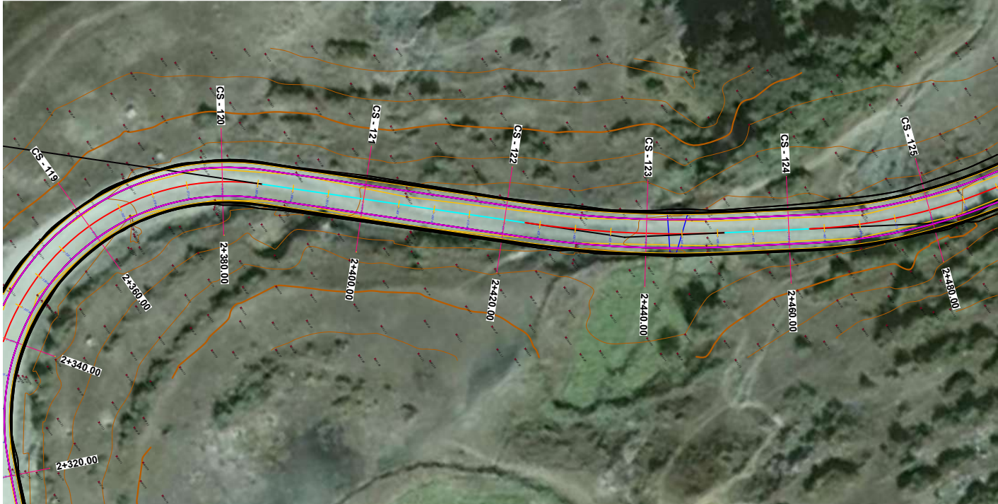
PLANIMETRIA DHE PROFILI GJATESOR I RRUGES SH 1:1000
