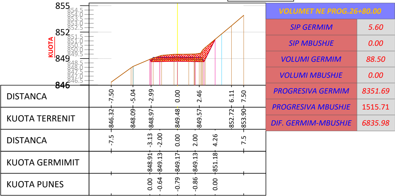
SC - 135 PROGRESIV. 2+680 m
