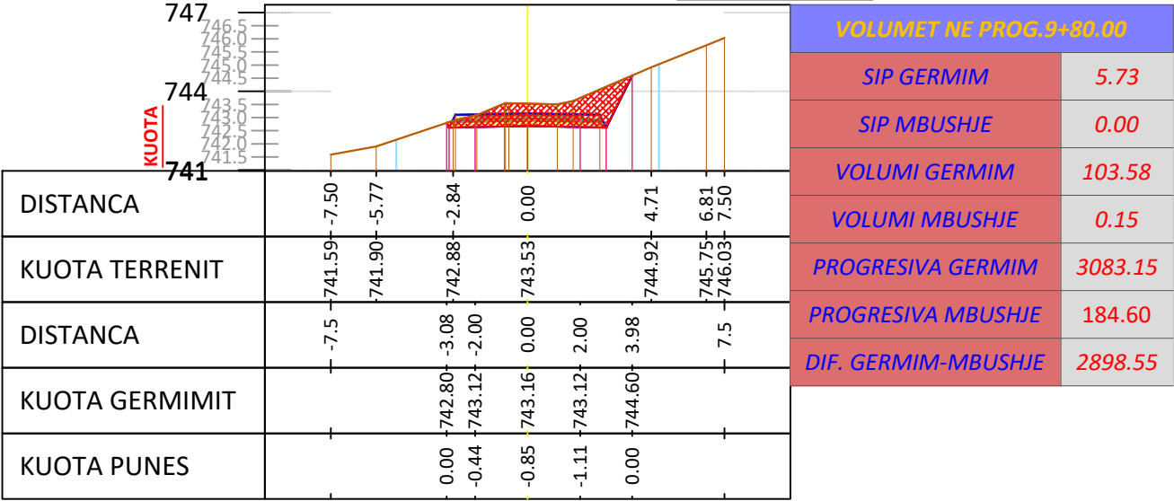
SC - 50 PROGRESIV. 0+980 m
