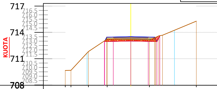
SC - 26 PROGRESIV. 0+500 m
