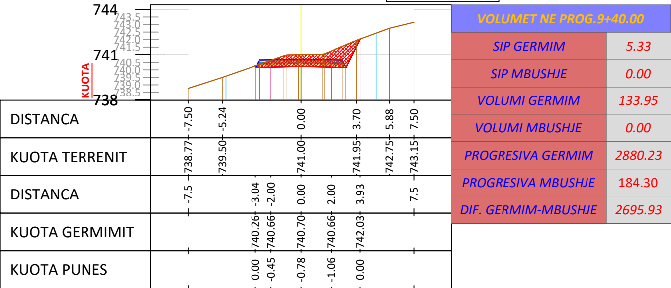
SC - 48 PROGRESIV. 0+940 m
