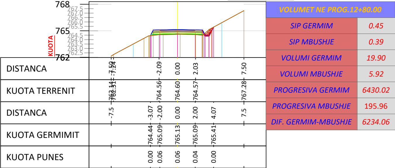
SC - 65 PROGRESIV. 1+280 m
