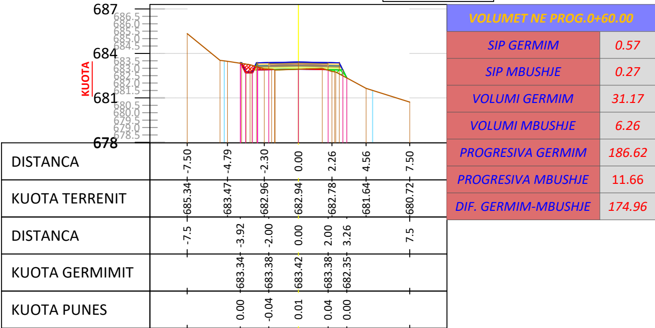
SC - 4 PROGRESIV. 0+060 m
