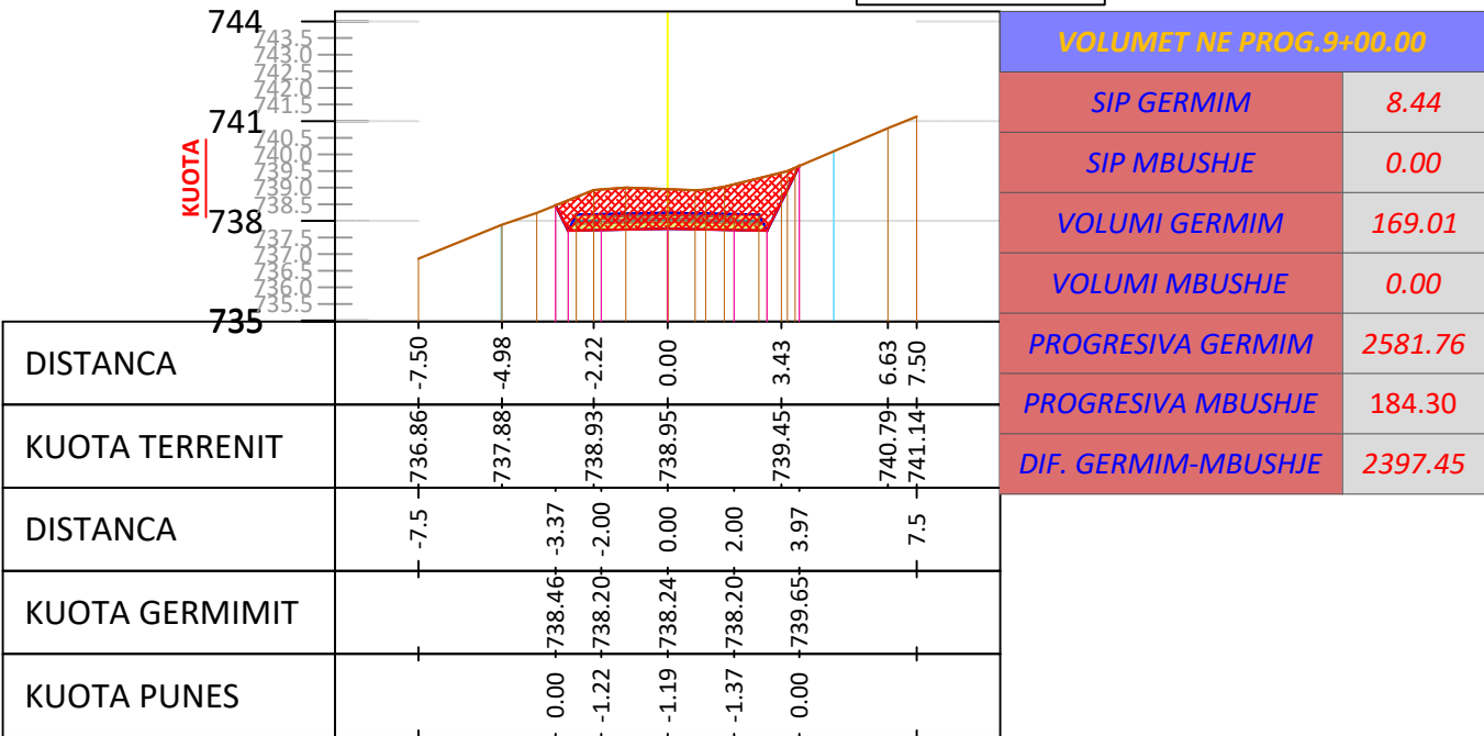
SC - 46 PROGRESIV. 0+900 m
