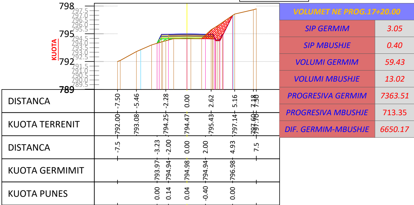
SC - 87 PROGRESIV. 1+720 m
