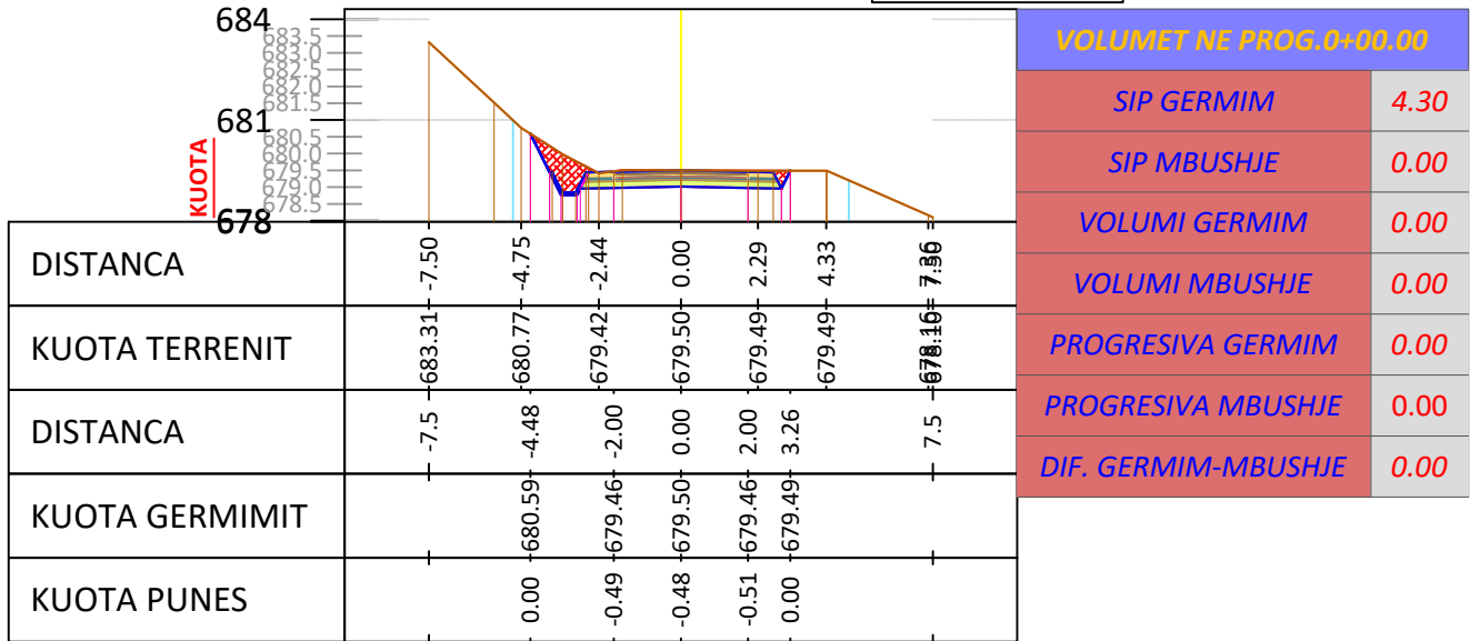
SC - 1 PROGRESIV. 0+000 m
