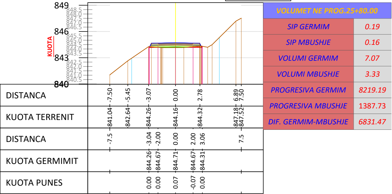
SC - 130 PROGRESIV. 2+580 m
