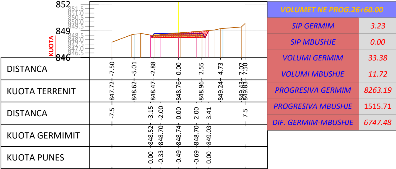
SC - 134 PROGRESIV. 2+660 m
