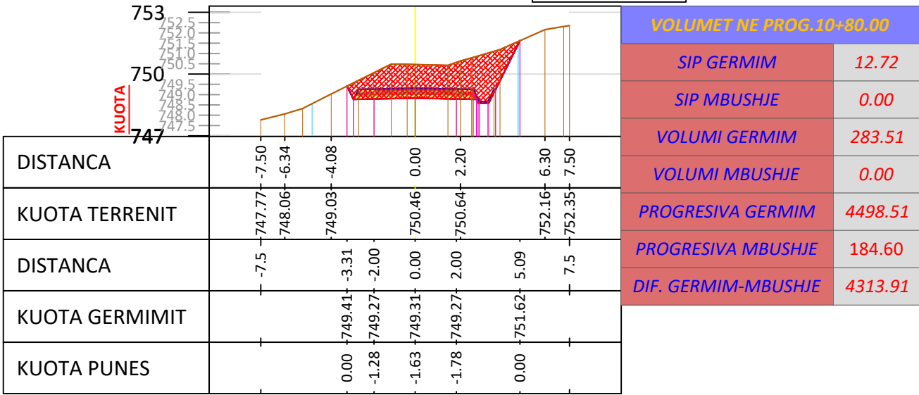
SC - 55 PROGRESIV. 1+080 m
