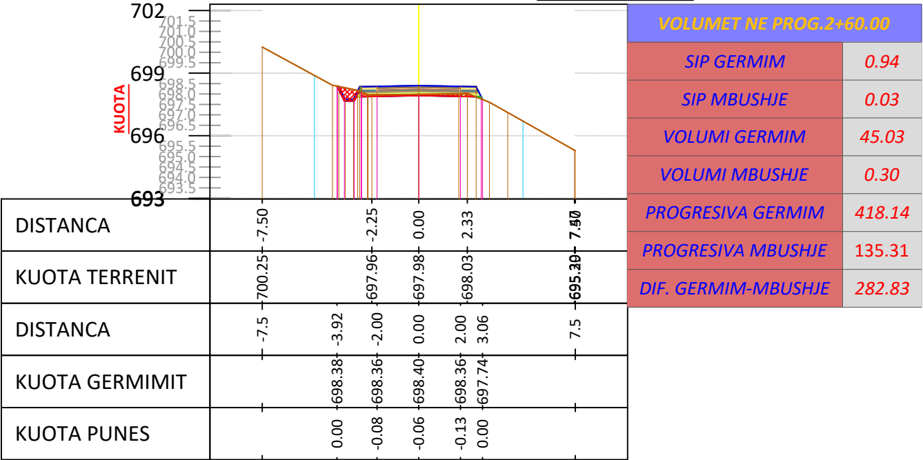
SC - 14 PROGRESIV. 0+260 m
