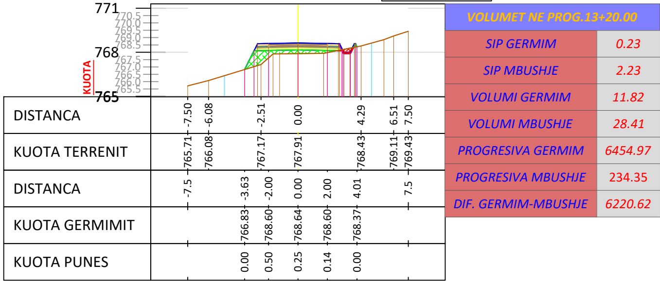
SC - 67 PROGRESIV. 1+320 m
