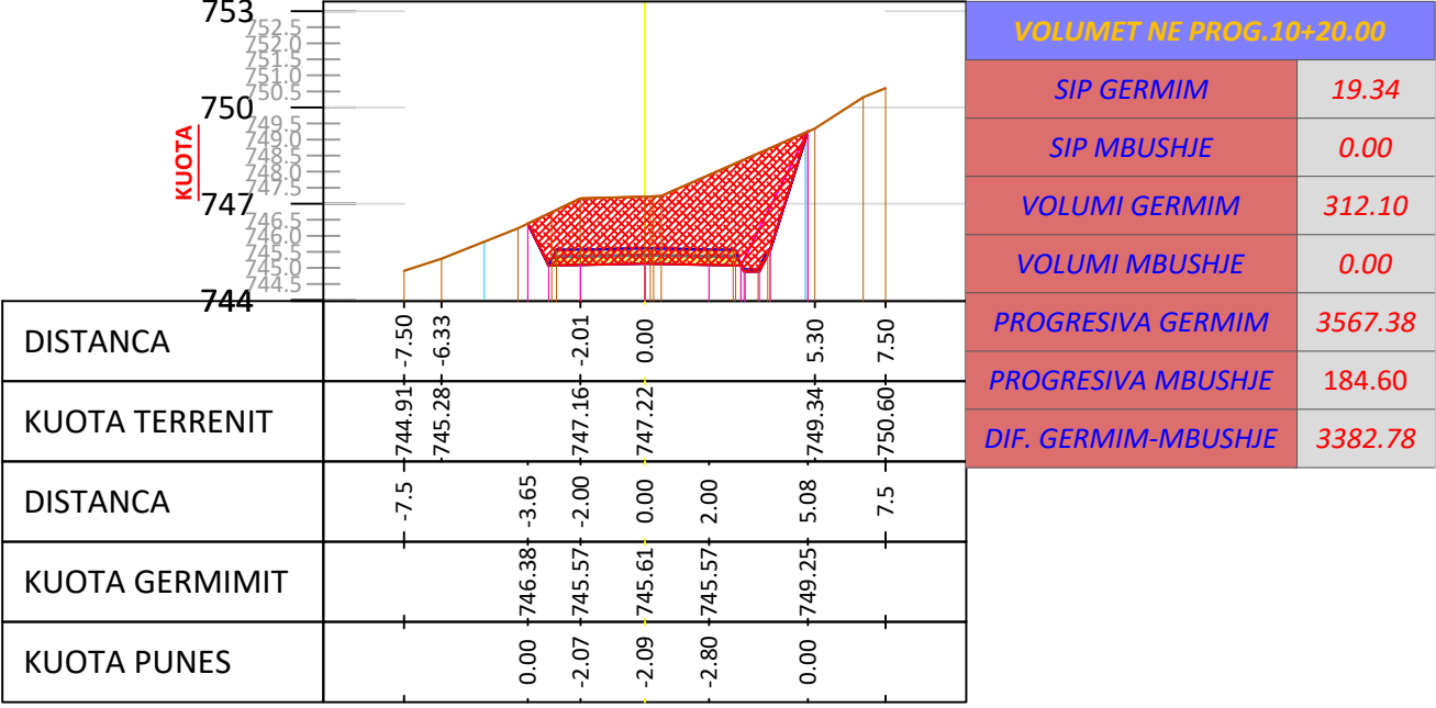
SC - 52 PROGRESIV. 1+020 m
