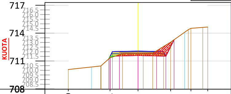
SC - 25 PROGRESIV. 0+480 m
