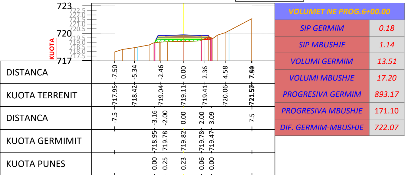
SC - 31 PROGRESIV. 0+600 m
