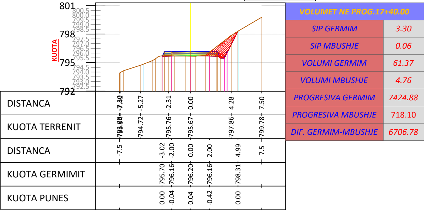
SC - 88 PROGRESIV. 1+740 m
