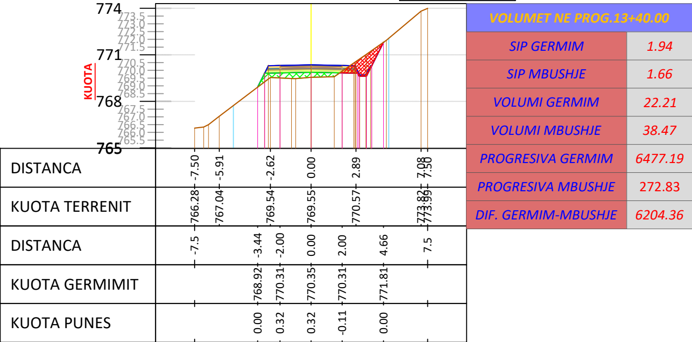
SC - 68 PROGRESIV. 1+340 m
