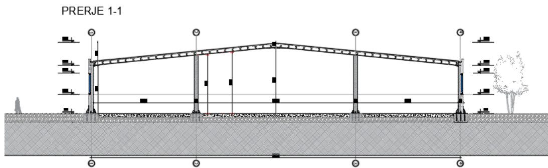
Figure 16. Prerja 1-1, Objekti i Perpunimit
