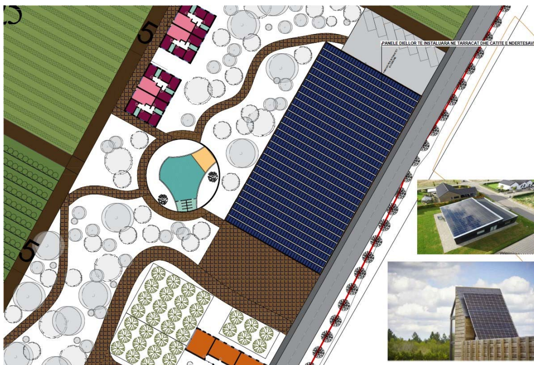
Figure 9. Panele diellore të instaluar në tarracat dhe çatitë e ndërtesave
