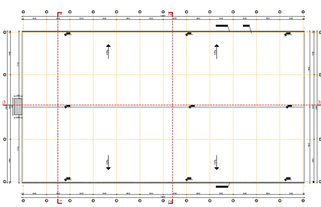
Figure 11. Plani i Catise, Objekti i Përpunimit
