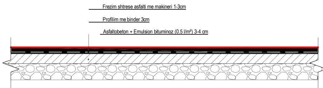
Figura 2-2: Profili tërthor tip B
