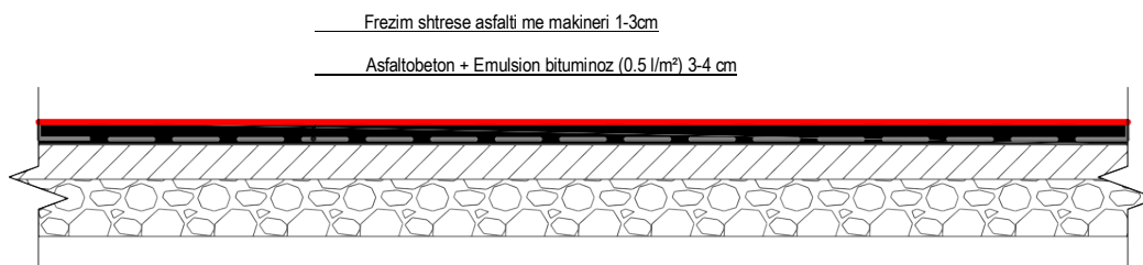
Figura 2-1: Profili tërthor tip A
