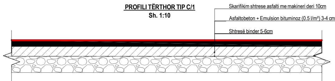
Figura 2-3: Profili tërthor tip C/1
