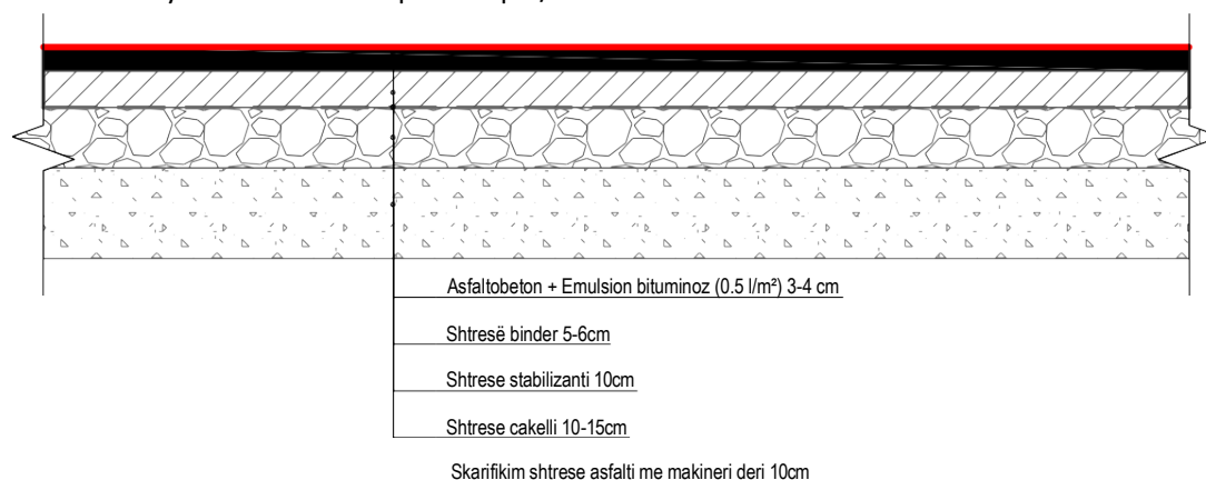
Figura 2-4: Profili tërthor tip C
