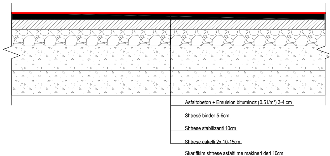
Figura 2-6: Profili tërthor tip E
