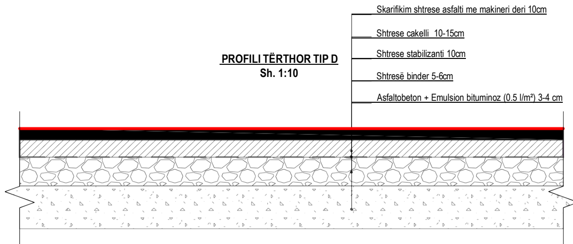
Figura 2-5: Profili tërthor tip D
