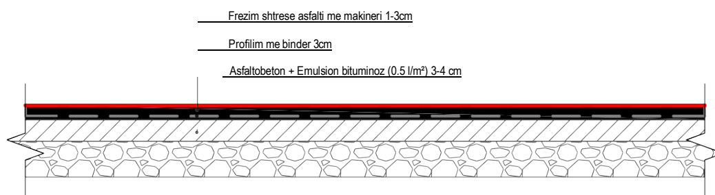
Figura 2-2: Profili tërthor tip B
