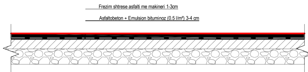
Figura 2-1: Profili tërthor tip A
