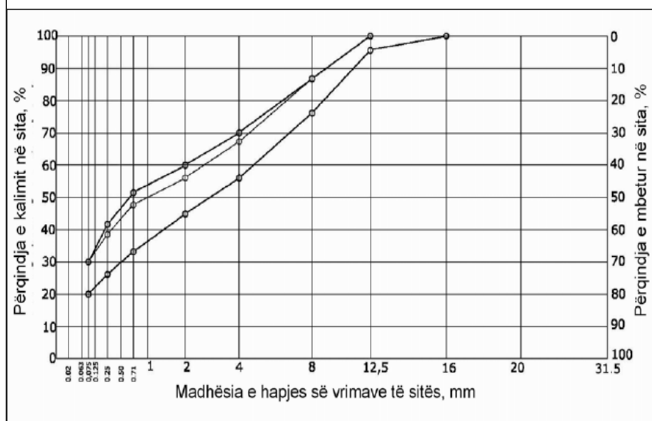
Figura 3.9: Kufinjët e kompozimit të përzierjeve të kokrrizave të gurit për ShSLS prej asfalti të rrjedhshëm ARr 12 dhe ARr 12S
