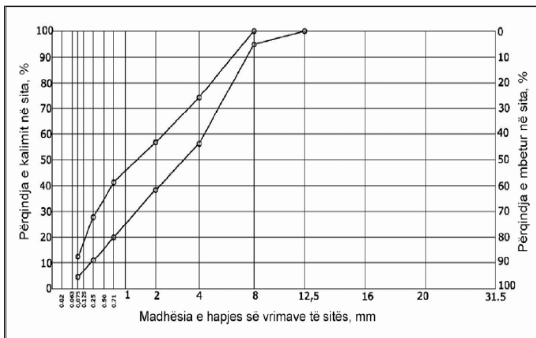
Figura 3.3: Kufinj të kompozimit të përzierjeve të kokrrizave të gurit për ShSLS prej asfaltobetoni të tipit AB 8
