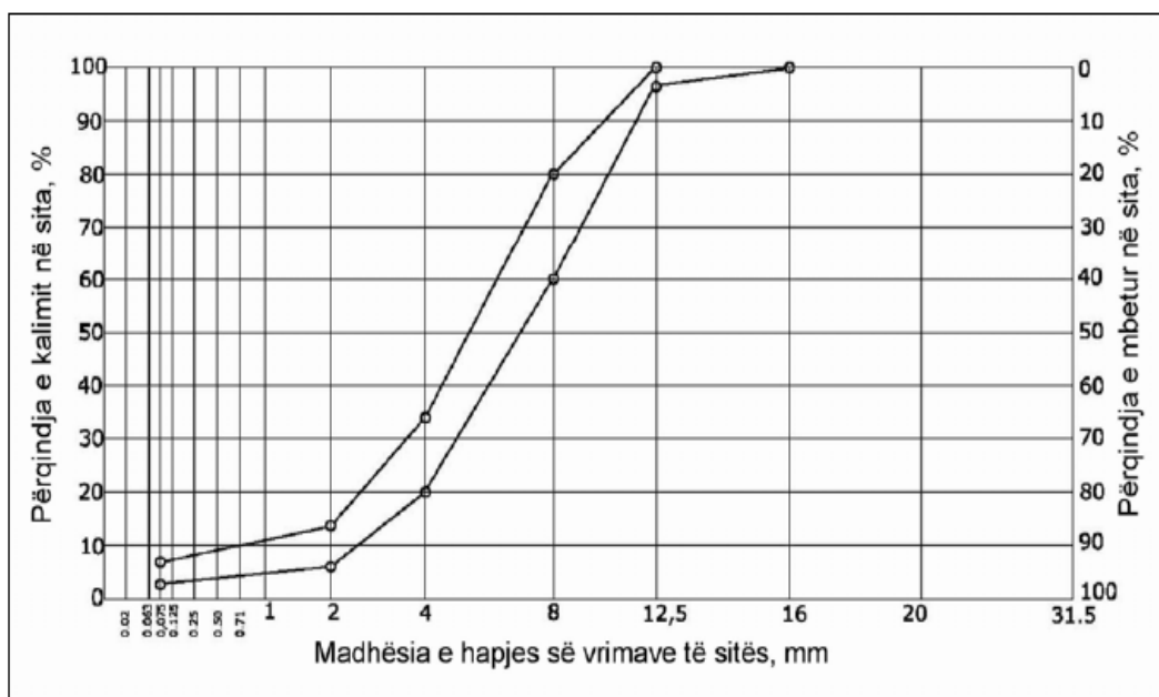
Figura 3.11: Kufinj të kompozimit të përzierjes së kokrrizave të gurit për ShSS prej përzierjeve të asfaltit poroz AP 12 dhe AP 12S
