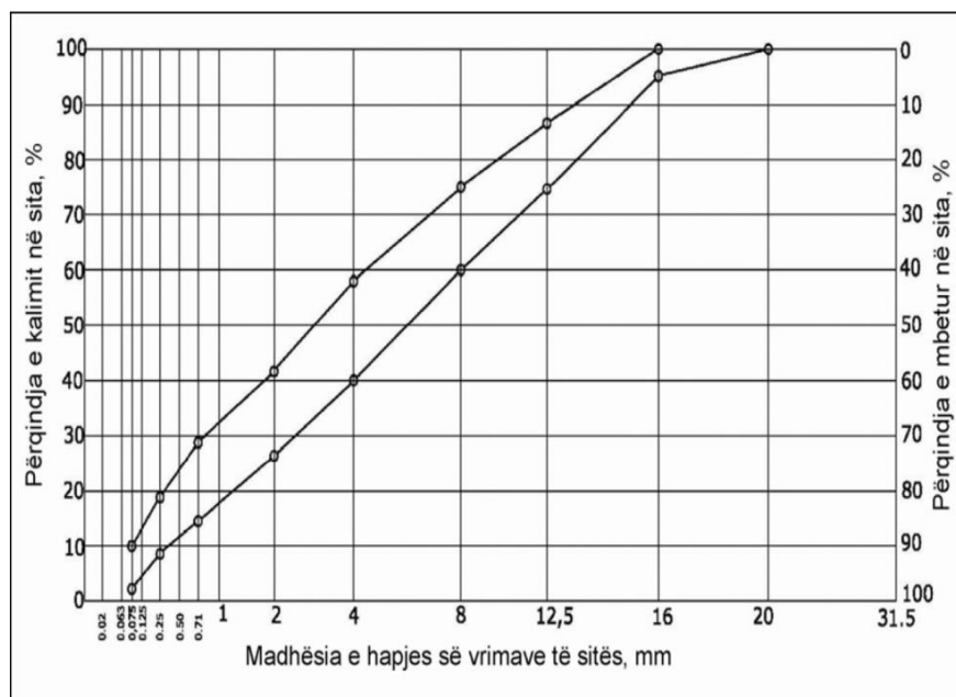
Figura 3.7: Kufinj të kompozimit të përzierjeve të kokrrizave të gurit për ShSLS prej asfaltbetoni të tipit AB 16. Së do përzierje e kokrrizave të gurit që parashikohet të përdoret për ShSLS, duhet të kontrollohet përpara fillimit të punimeve në përputhje me kërkesat e këtyre kushteve teknike. Numri i mostrave do të përcaktohet nga Inxhinjeri Mbikqyrës. Përsëritja e kontrollit nuk është e nevojshme të kryhet për rastet kur Inxhinjeri Mbikqyrës ka dhënë tashmë miratimin ndaj Kontraktorit për përdorimin e një përzierjeje të njëjtë të kokrrizave të gurit për t'u vendosur në ShSLS.
