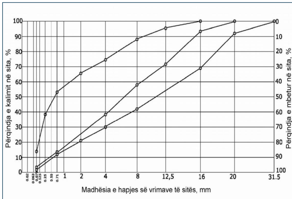
Figura 2.7: Kufinjtë e formimit të përzierjeve prej materiali të granular të kokrrizave të gurit për bazat bituminoze të rrugës Zh1B 16 dhe Zh1BÇGTh 20
