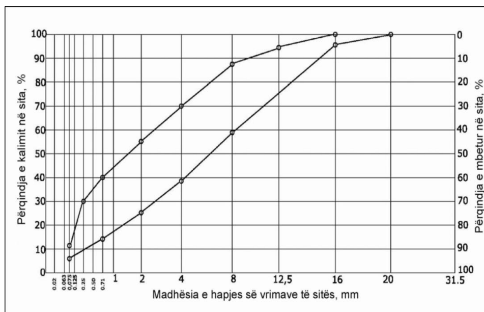
Figura 2.13: Kufinj të formimit të përzierjeve prej materiali të granular të kokrrizave të gurit për bazën prej makadami bituminoz - MB 22
