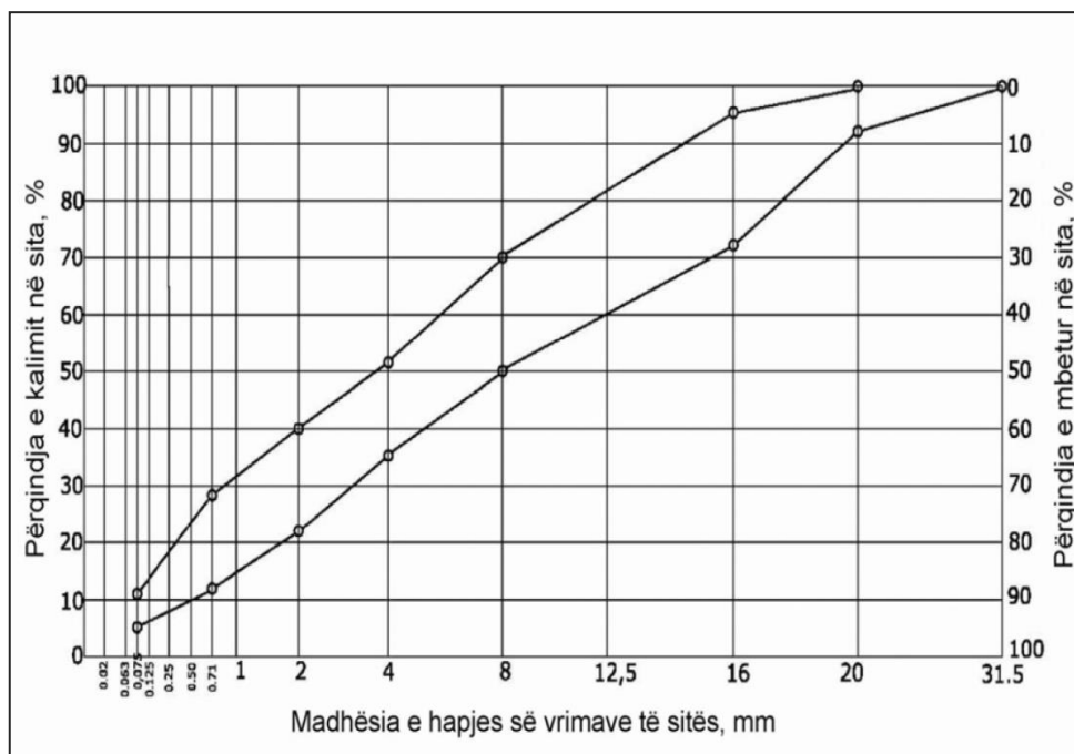
Figura 2.8: Kufinjtë e formimit të përzierjeve prej materiali të granular të kokrrizave të gurit për bazën bituminoze të rrugës Zh1BÇGTh 20S
