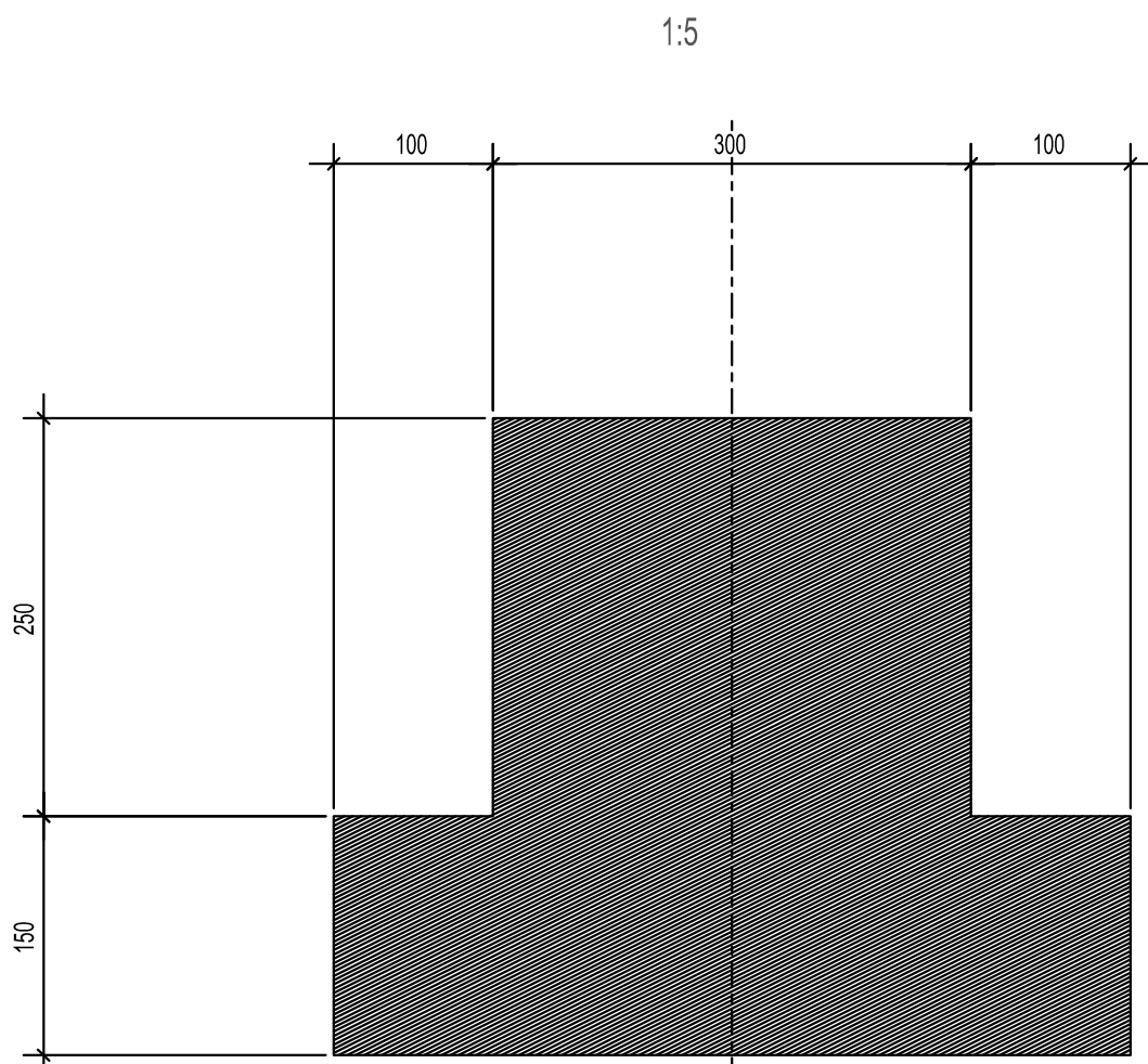
trau T lidhes midis kolonave
