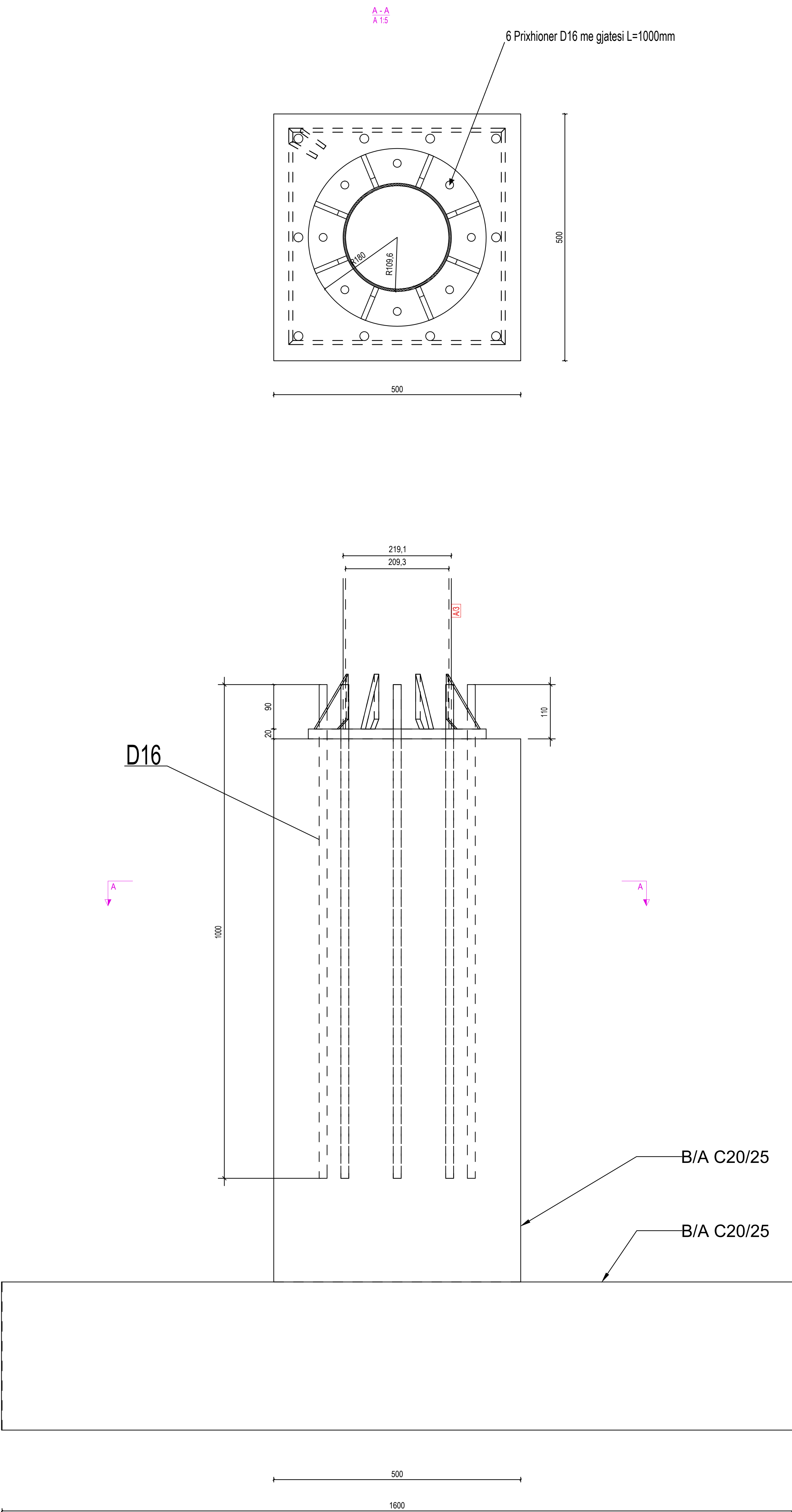
Detaji i prirhionereve
