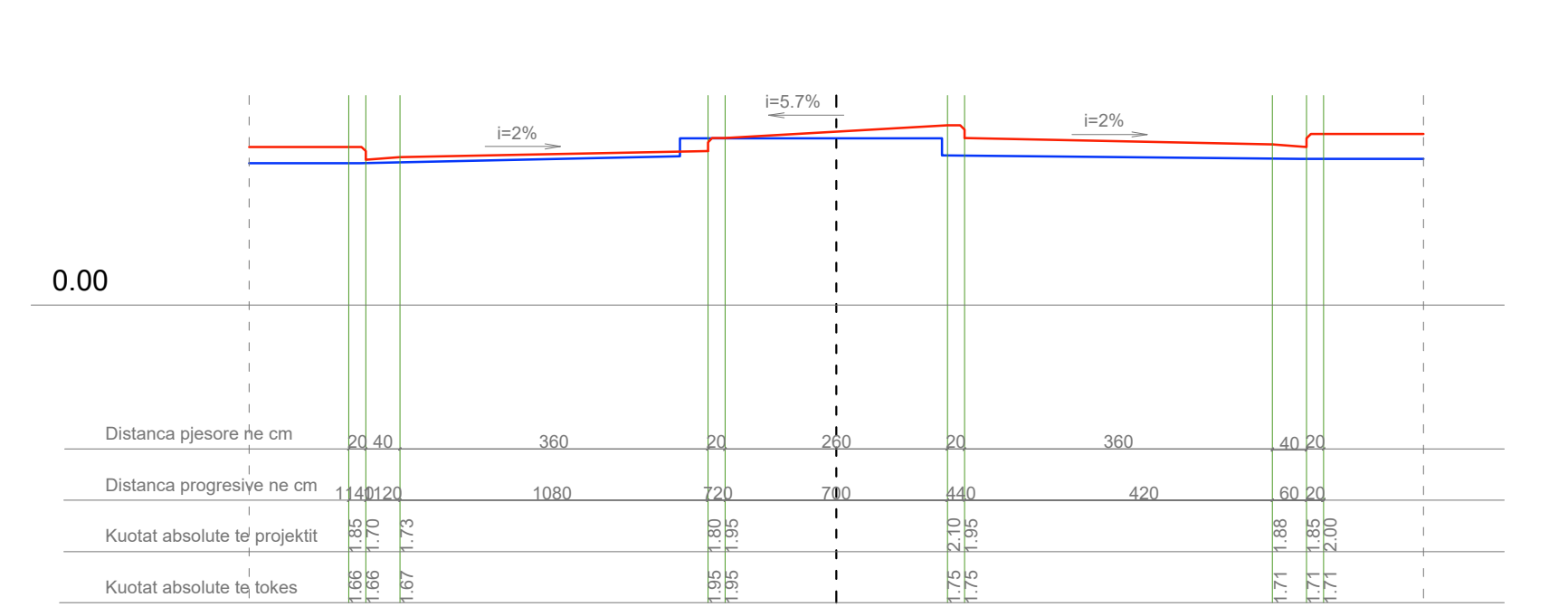
Prerja 9-9
