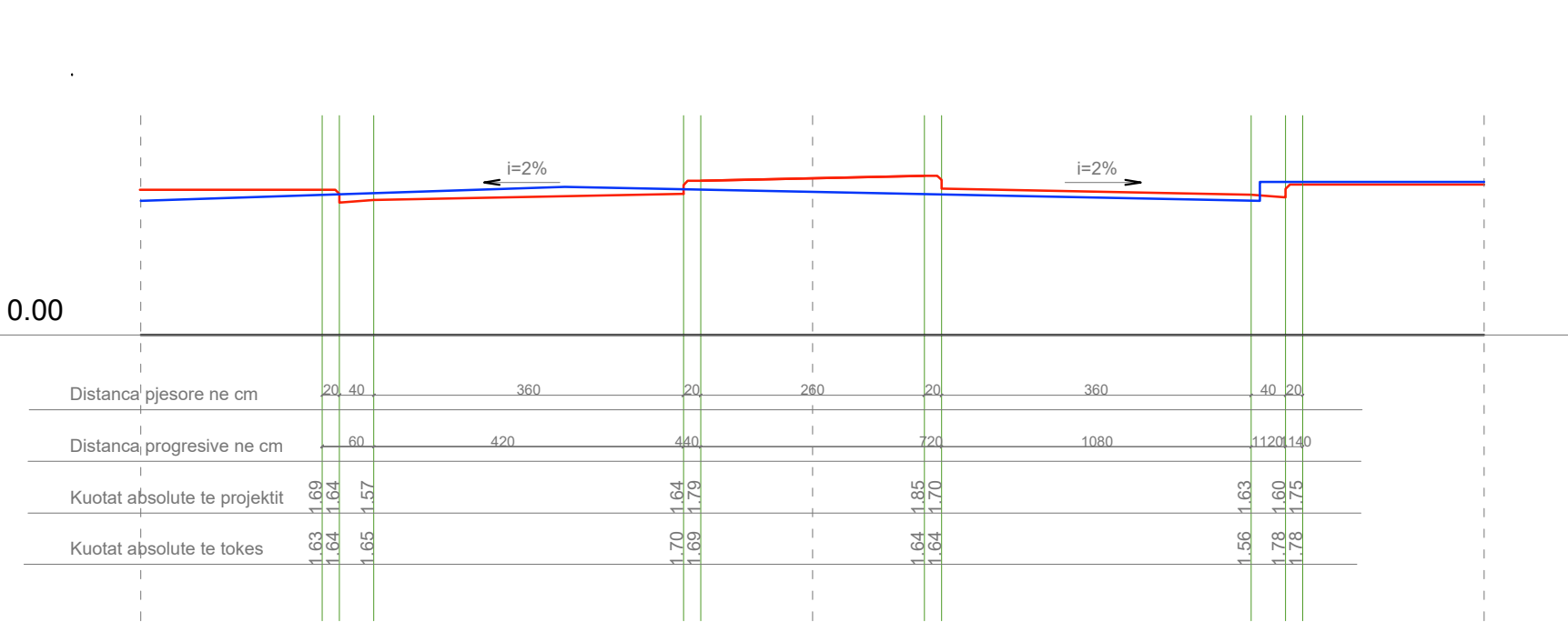
Prerja 4-4
