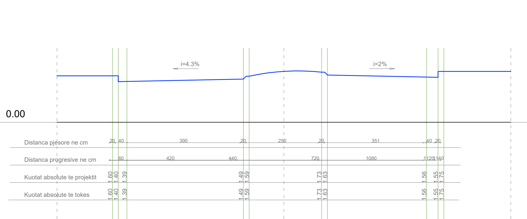
Prerja 1-1
