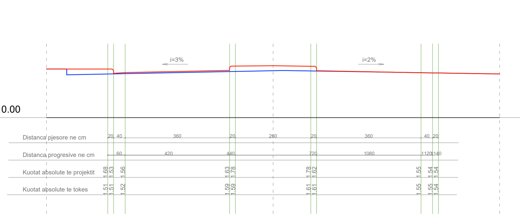
Prerja 2-2
