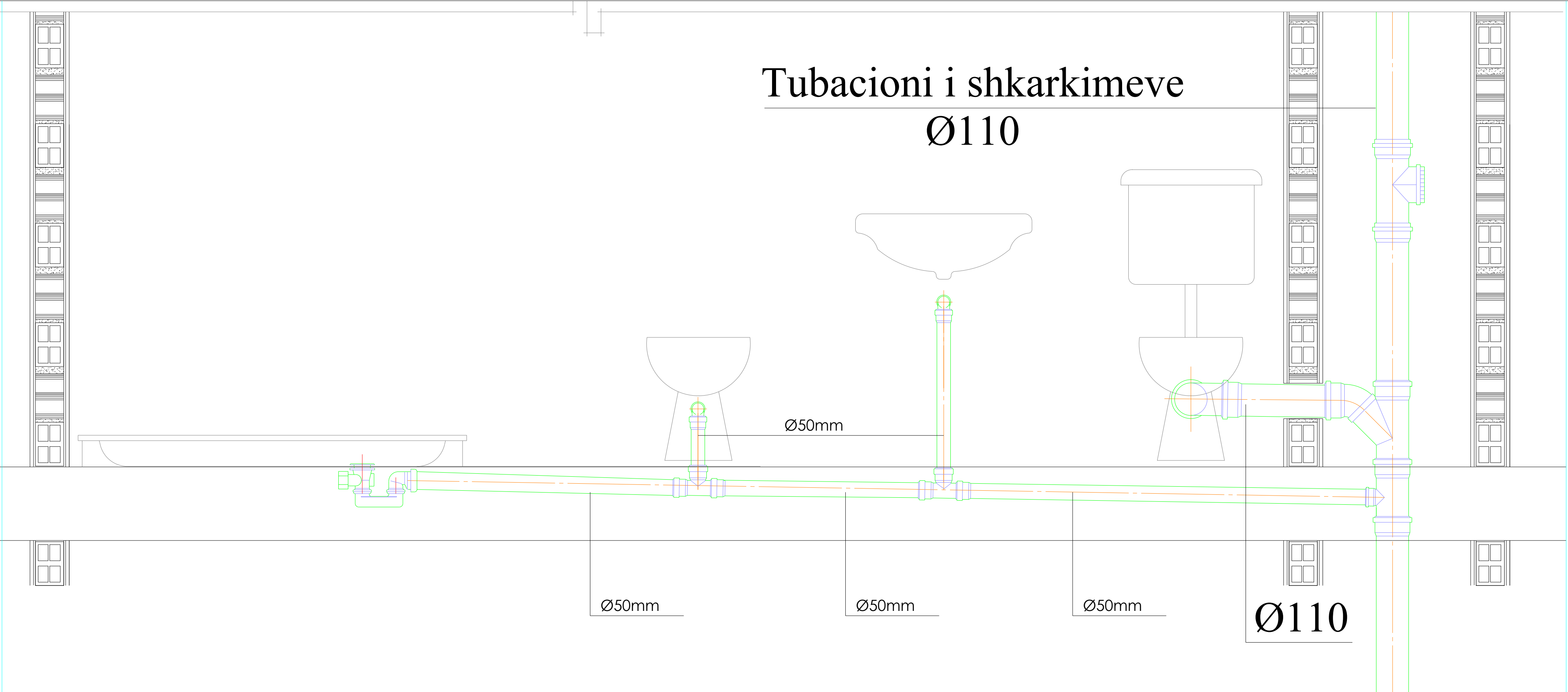
LIDHJA E PAJISJEVE SANITARE ME KOLONAT E SHKARKIMEVE
