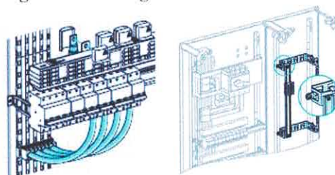
Figura 2 : Kite të gatshme dhe aksesore të nevojshëm
