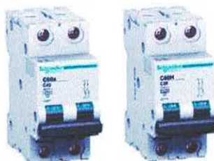
Figura 5 : Automatë dy polarë sipas CEI 60947-2
