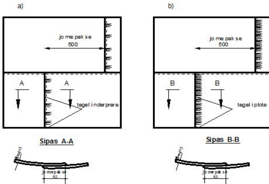
Konstruksioni i tegelave vertikale i montuar njeri mbi tjetrin
