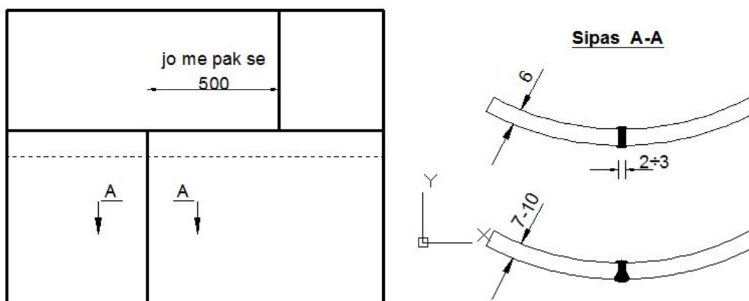
Konstruksioni i tegelit vertikal i montuar koke me koke
