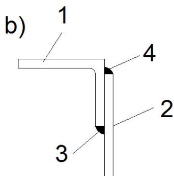
b) Konstruksioni i bashkimit te angolarit te siperm unazor
