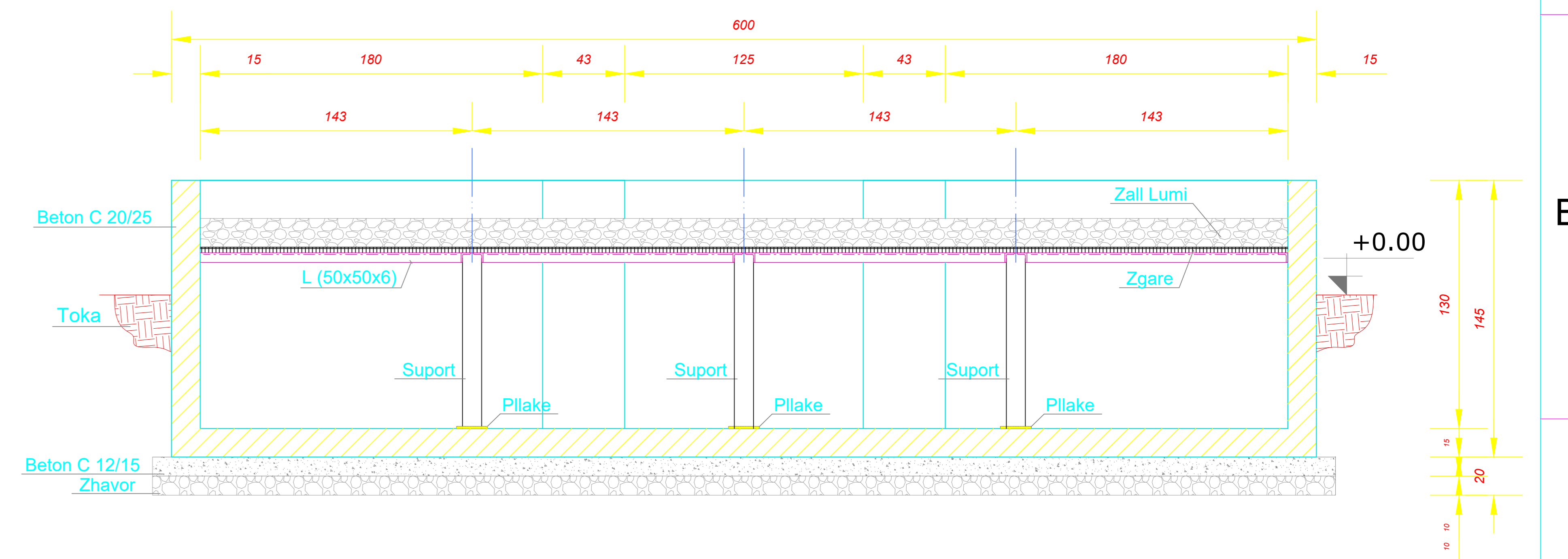
Prerja C - C
