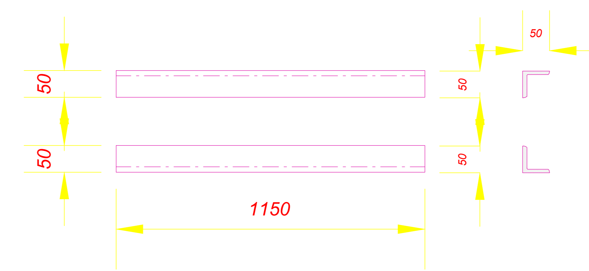
Poz. 3 L 50x50x6 (2 copë)
