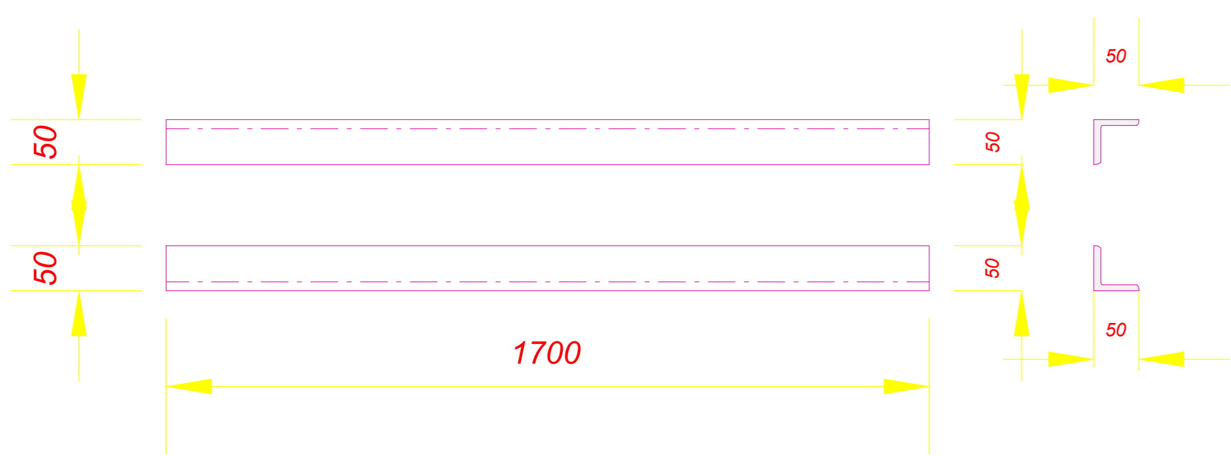
Poz. 2 L 50x50x6 (4 copë)
