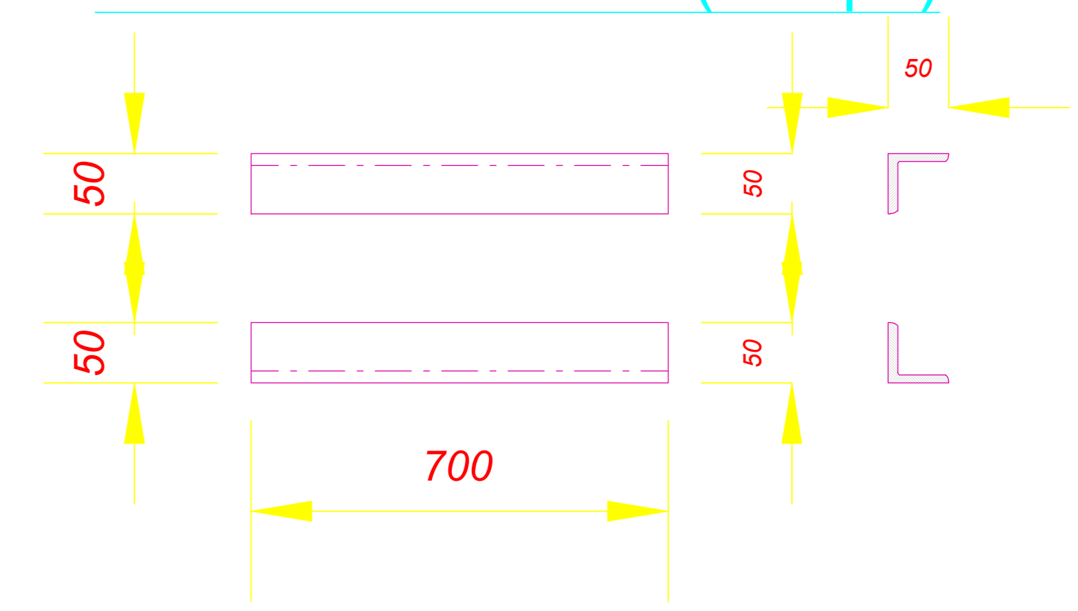
Poz. 7 L 50x50x6 (8 copë)
