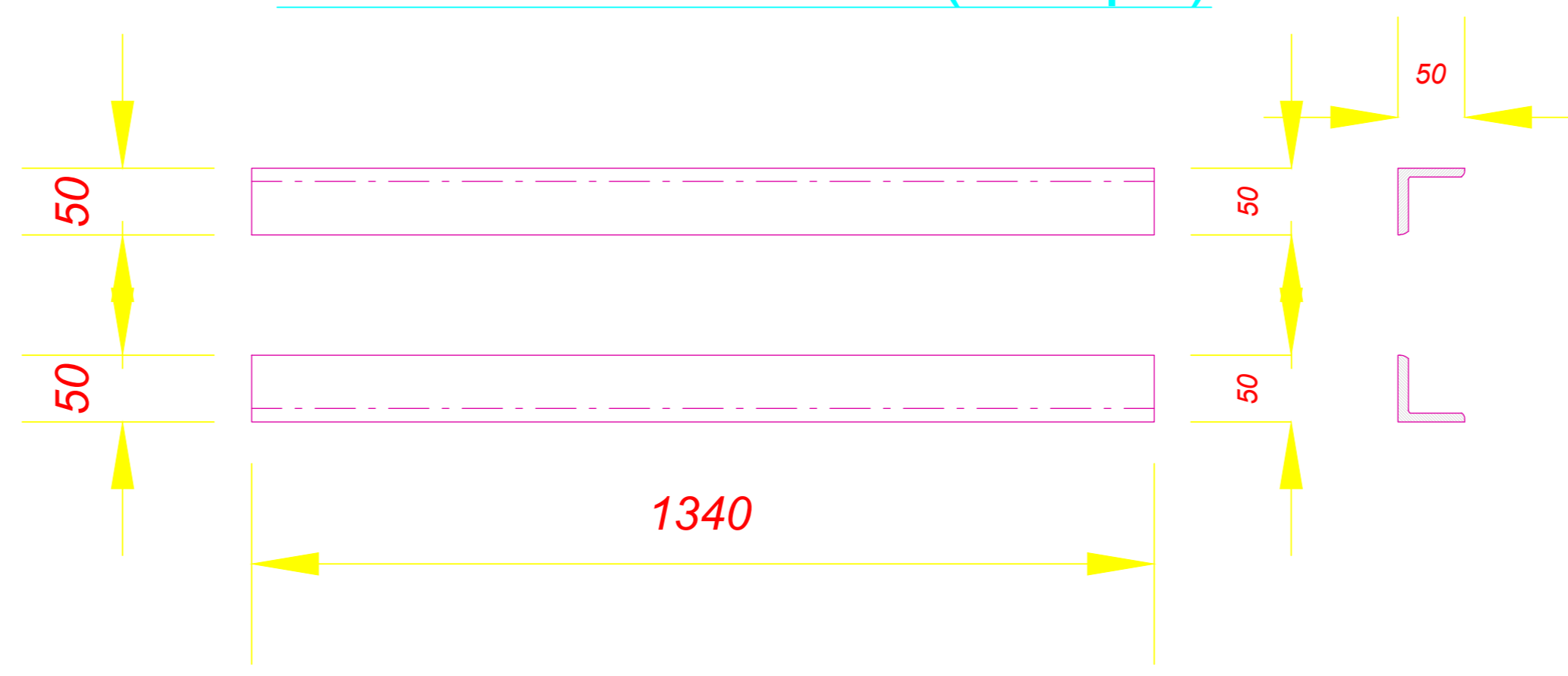
Poz. 5 L 50x50x6 (2 copë)
