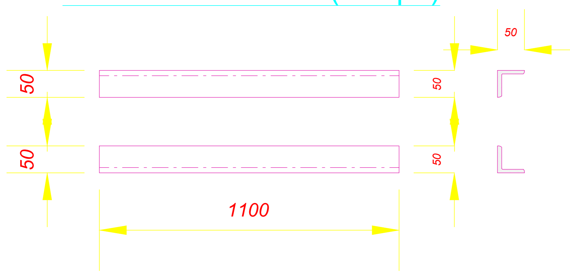
Poz. 4 L 50x50x6 (2 copë)
