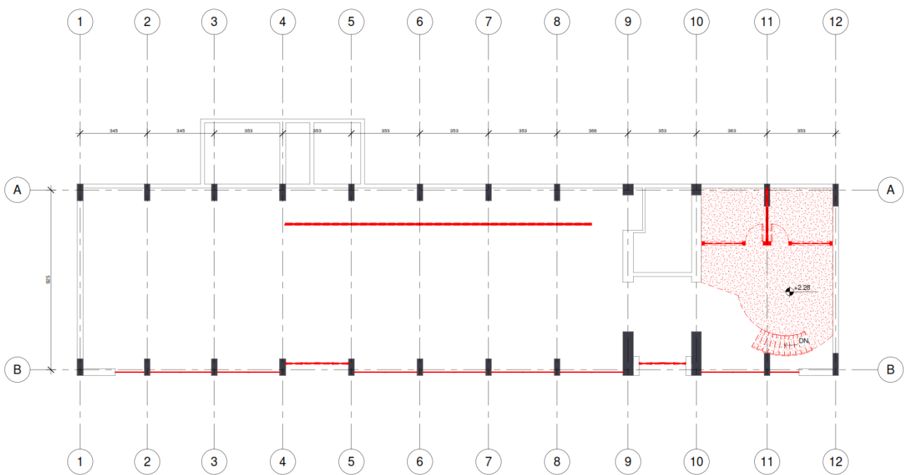
Plani i prishjeve ne nderkat
