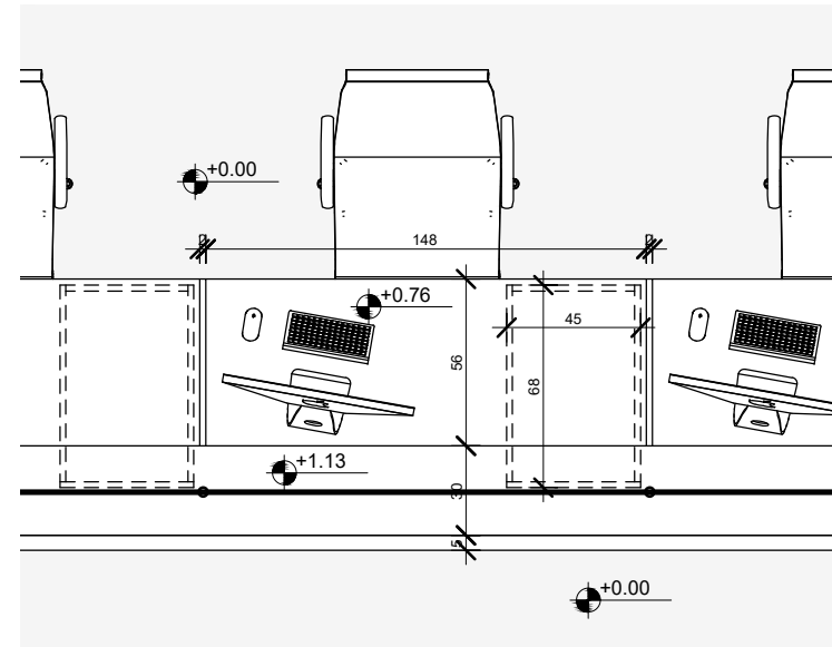
3 tavoline pune plan 1 : 20
