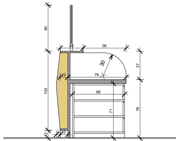
1 tavoline pune prerje 1 : 20
