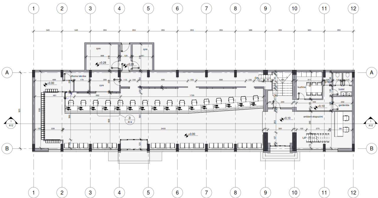
Planimetria e katit perdhe
