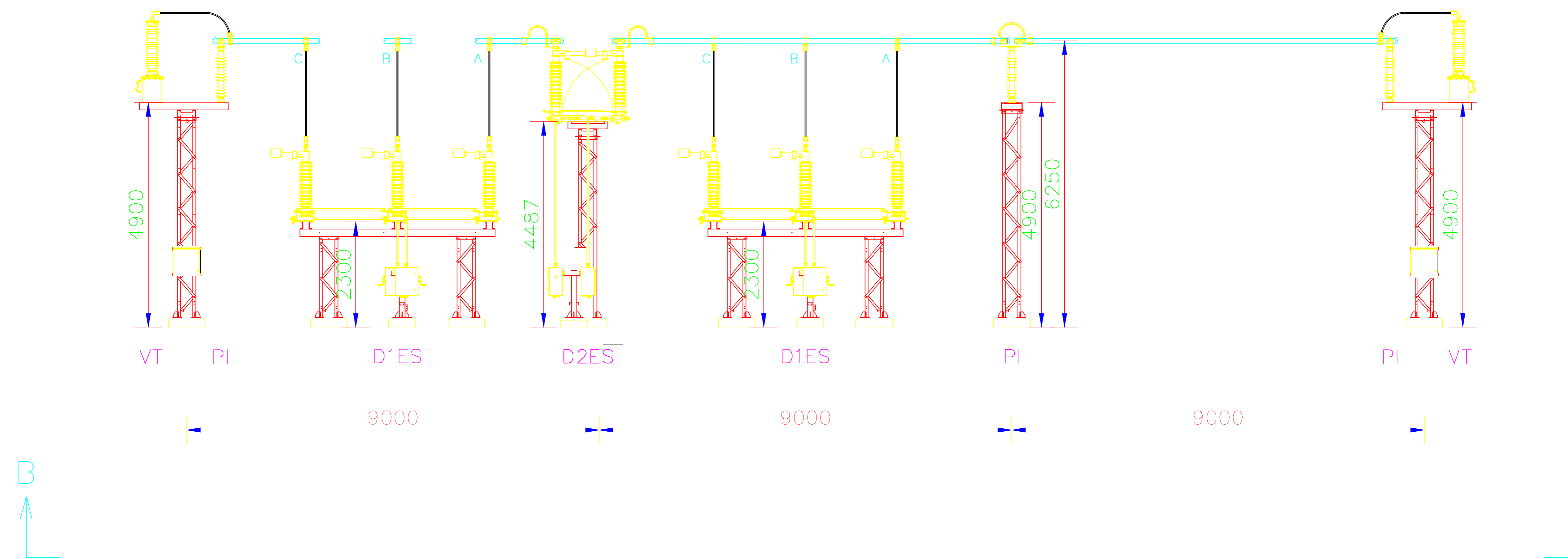
Prerja tërthore e zbarrave 110kV
