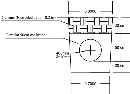
Germim kanali - Tubi Ø400mm
