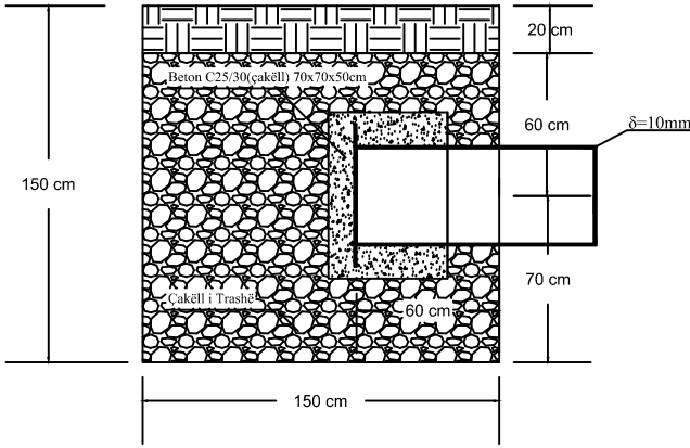
Gropa e operimit 1.5m x1.5m x1.5m (2 cope) (Gjatesia e kanalit te tubacionit 400 mm = 825 ml)
