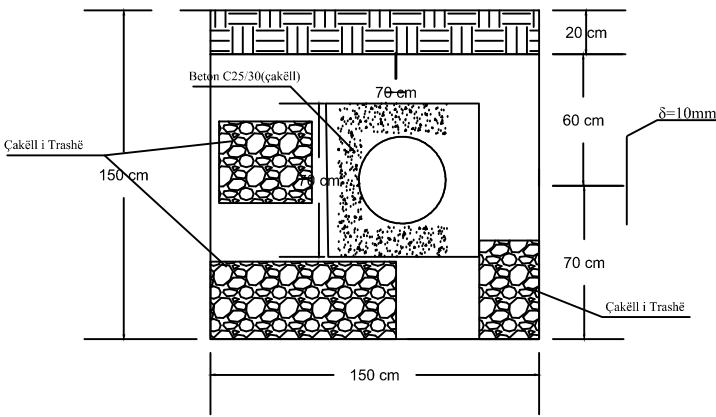
Gropa e operimit (1.5x1.5x1.5) m (2 cope)
