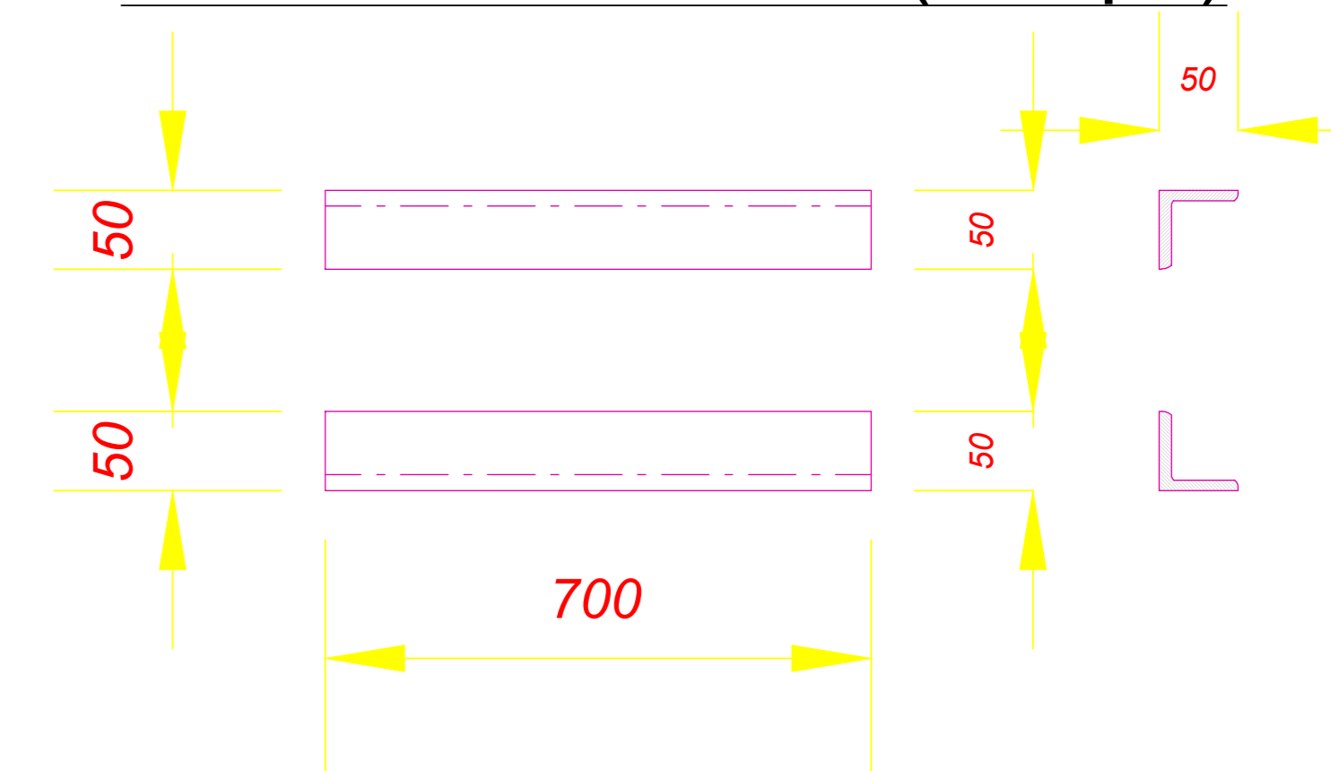
Poz. 7 L 50x50x6 (8 copë)
