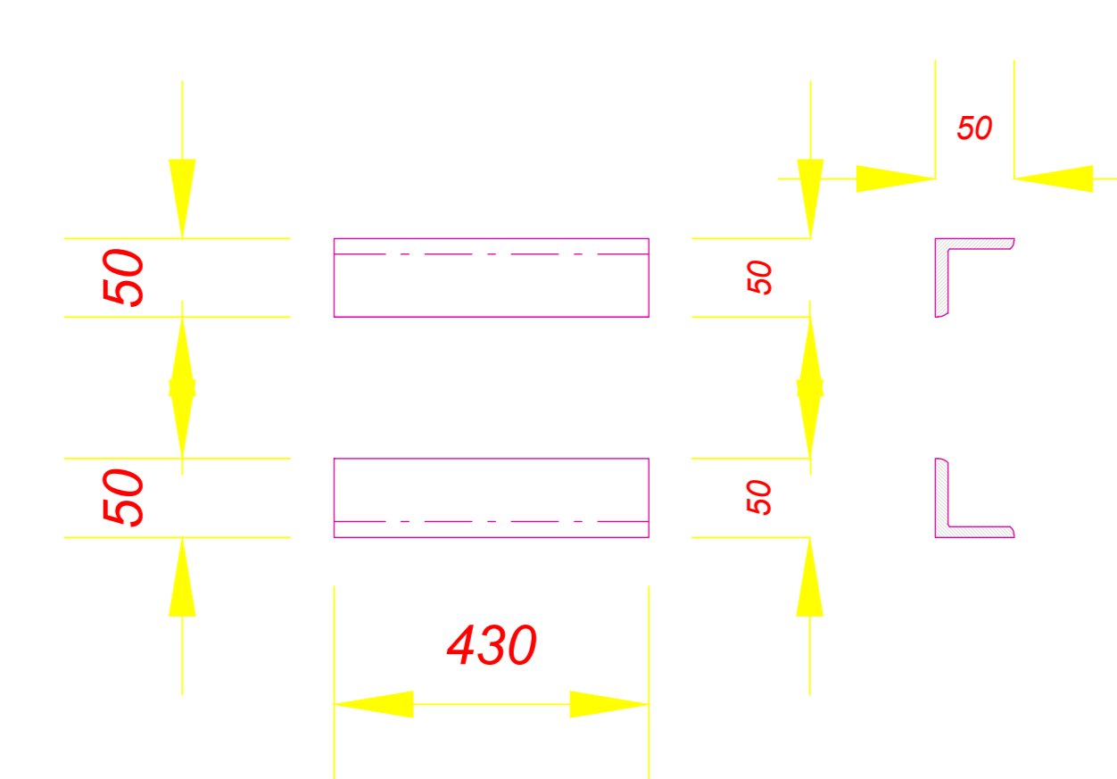
Poz. 8 L 50x50x6 (4 copë)
