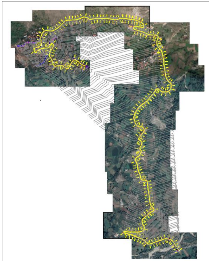
Horografia e Rruges Shengjin deri ne fshatin Shen Meri
