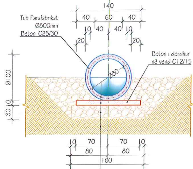
PRERJA A-A, Sh. 1:50
