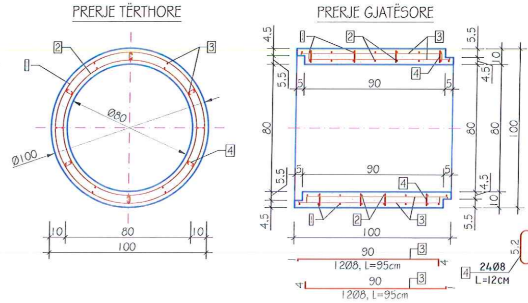
ARMATURA SPIRALE PER D=80cm
