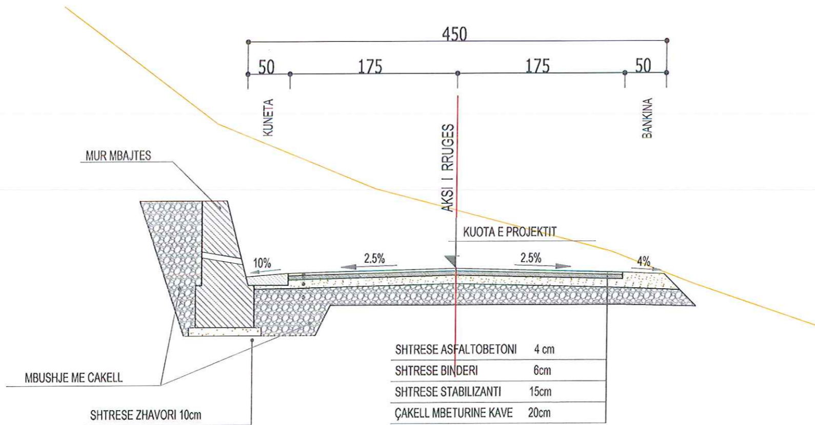
PROFIL TERTHOR TIP 5
