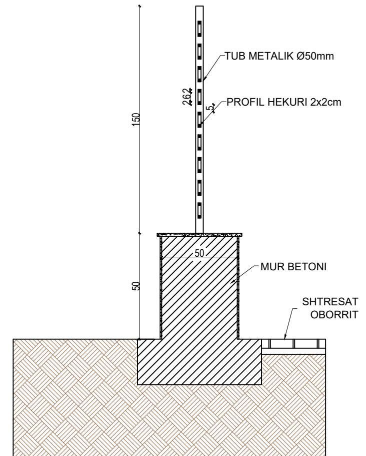
PRERJE 1-1 Sh 1:25
