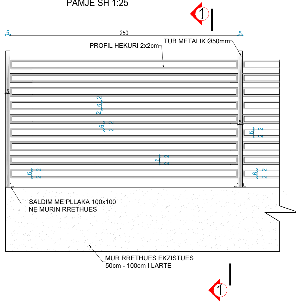
PAMJE SH 1:25
