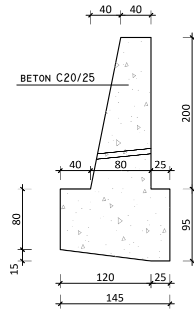
Mur prites C20/25 h=2.0m Sh 1:50
