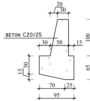
Mur prites C20/25 h=1.0m Sh 1:50
