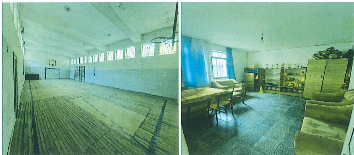
Foto te gjendjes ekzistuese te palestres
