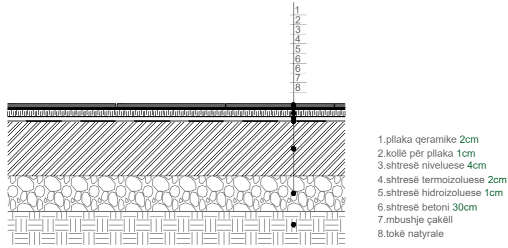
D1: SHITESAT E DYSHEMESË / KATI PËRDHE / sh. 1:15
