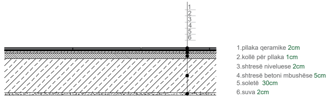
D2: SHITESAT E DYSHEMESË / KATI +1,+2 / sh. 1:15
