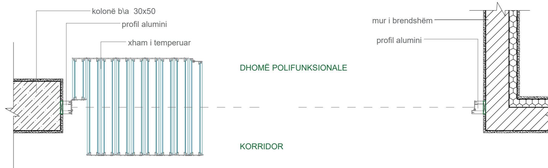
D8: DETAJ I VETRATËS SË PALOSSHME | PLAN sh. 1:10
