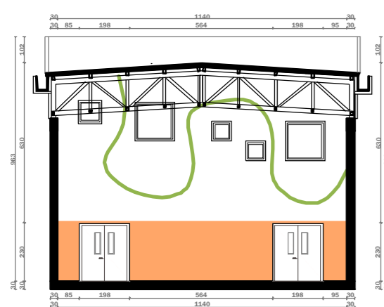
Pamja 06 Shkalla 1:150
