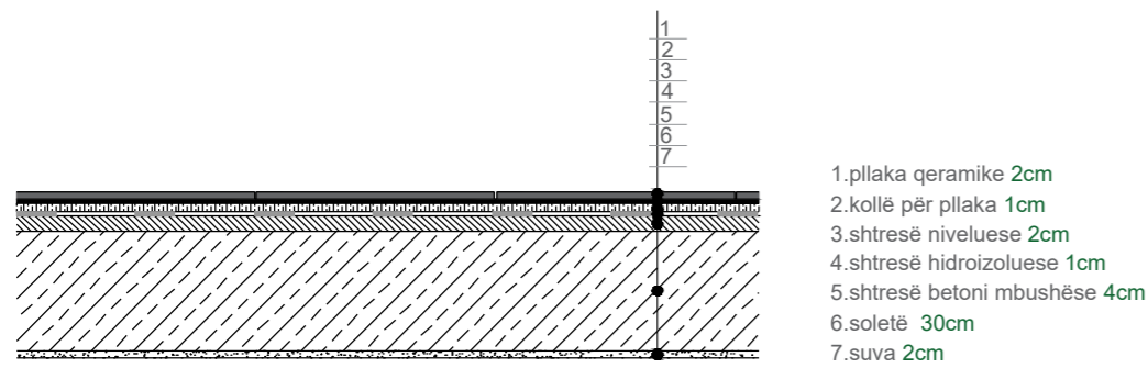
D3: SHITESAT E DYSHEMESË / TUALETET / sh. 1:15
