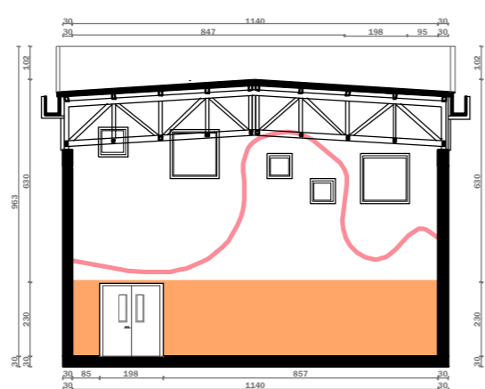
Pamja 05 Shkalla 1:150
