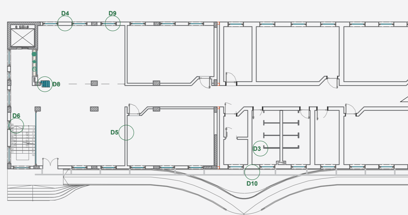
PLAN I KATIT PËRDHE EVIDENTIMI I DETAJEVE 1:200
