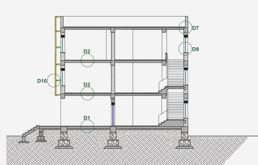
PRERJE A-A EVIDENTIMI I DETAJEVE 1:200
