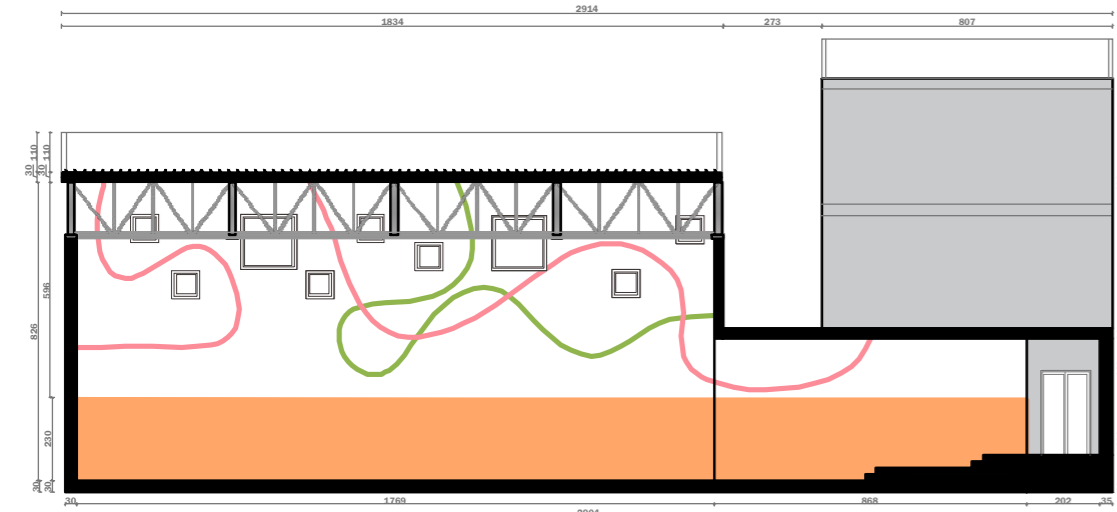
Pamja 08 Shkalla 1:150
