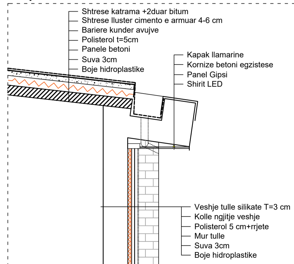
Detaj 1
