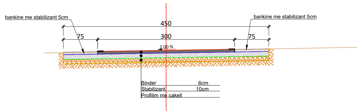
Profil Tip 1 "Segmenti SHKOZË" Km 0+000.00 - 0+700.00
