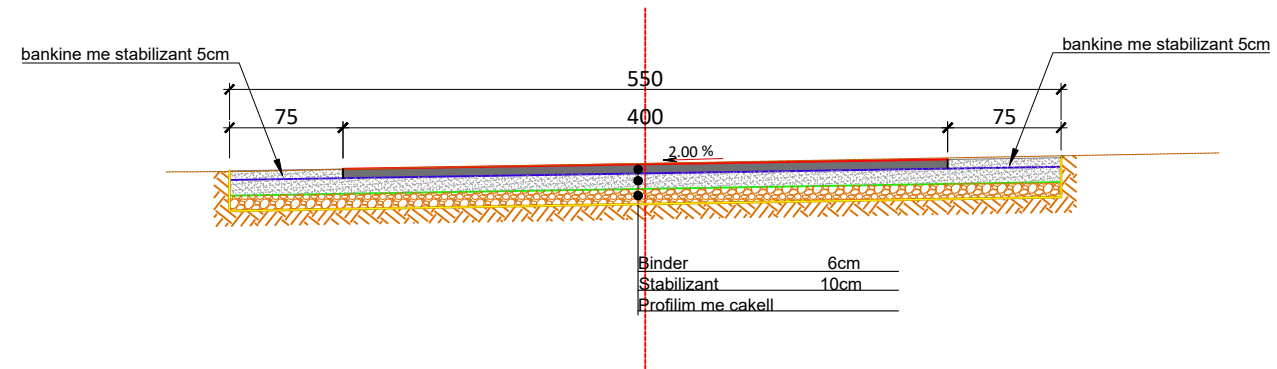
Profil Tip 1 "Segmenti IDRIZ" Km 0+000.00 - 1+000.00
