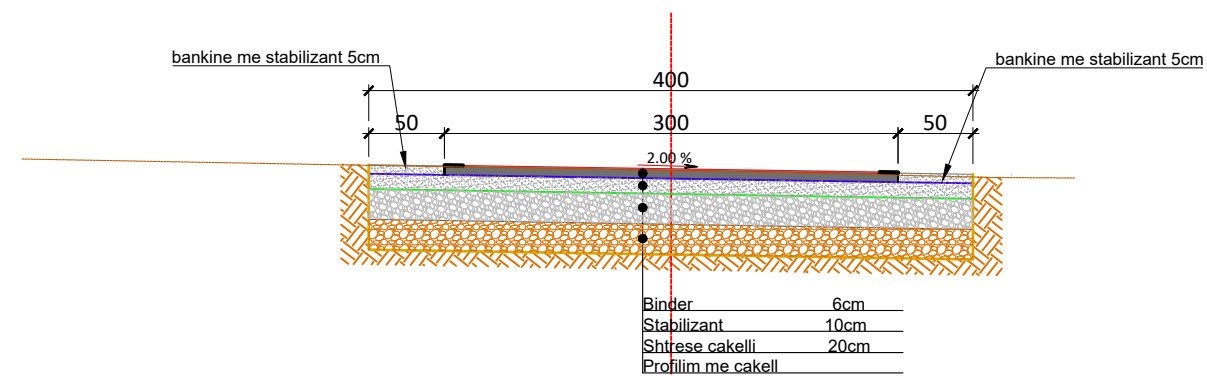
Profil Tip 1 "Segmenti Seferan"
