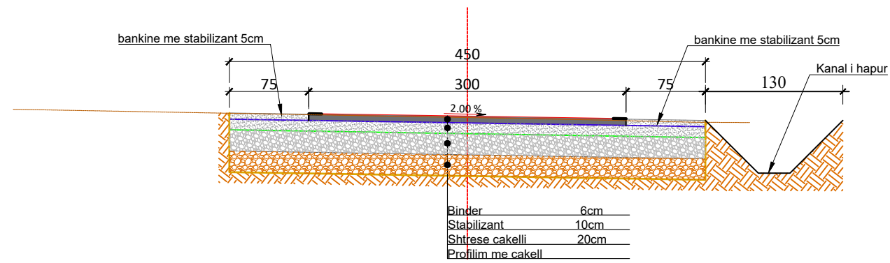
Profil Tip 2 "Segmenti SHKËNDI"
