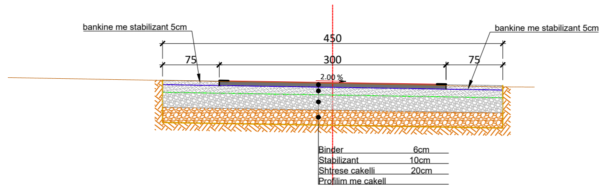
Profil Tip 1 "Segmenti SHKËNDI"
