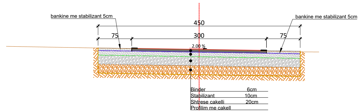
Profil Tip 1 "Segmenti TURBULL"
