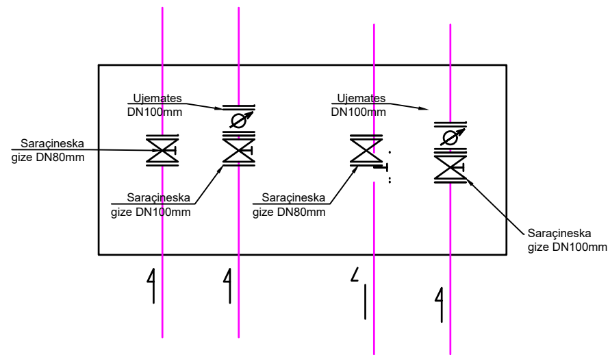
SKEMAT E PUSITES EKZISTUESE P20,P21,P22 PAS NDERHYRJES
