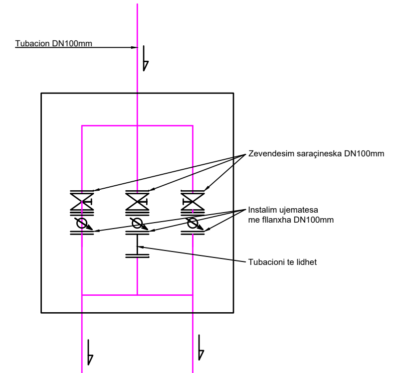
SKEMAT E PUSITES EKZISTUESE P17,P18,19 (E PERFUNDUAR)
