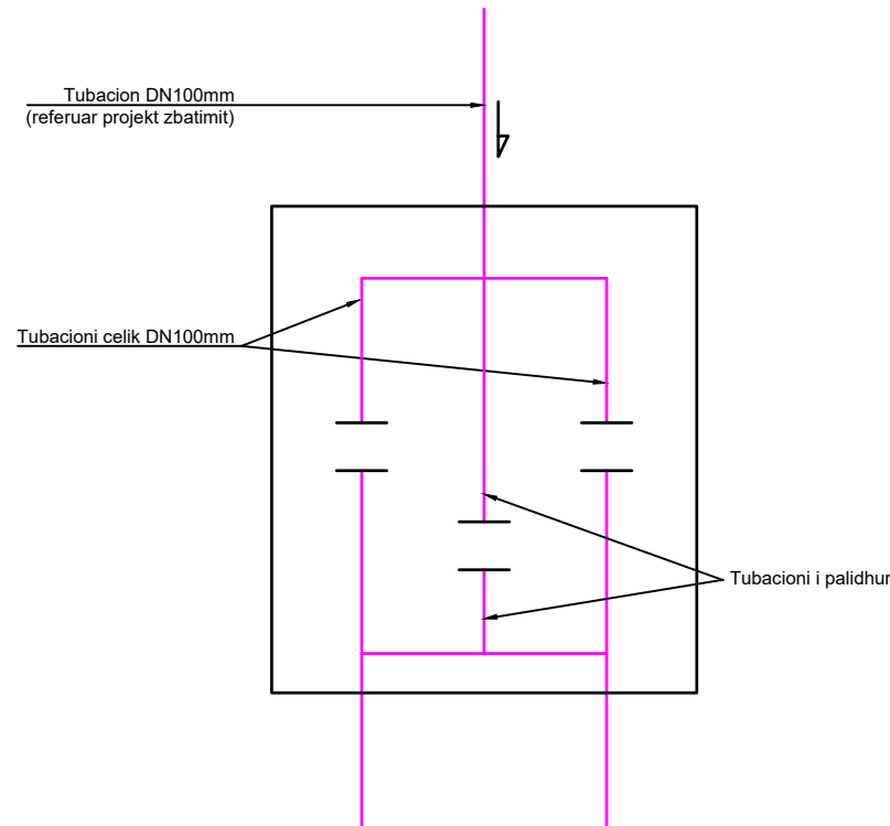
SKEMAT E PUSITES EKZISTUESE P17,P18,19 (PUSETE FURNIZIM REZERVUARIT) SIPAS VERIFIKIMIT NE VEND
