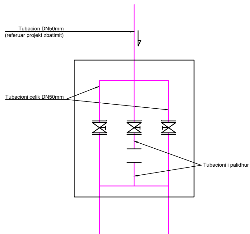
SKEMAT E PUSITES EKZISTUESE P2 (PUSETE FURNIZIM REZERVUARIT) SIPAS VERIFIKIMIT NE VEND
