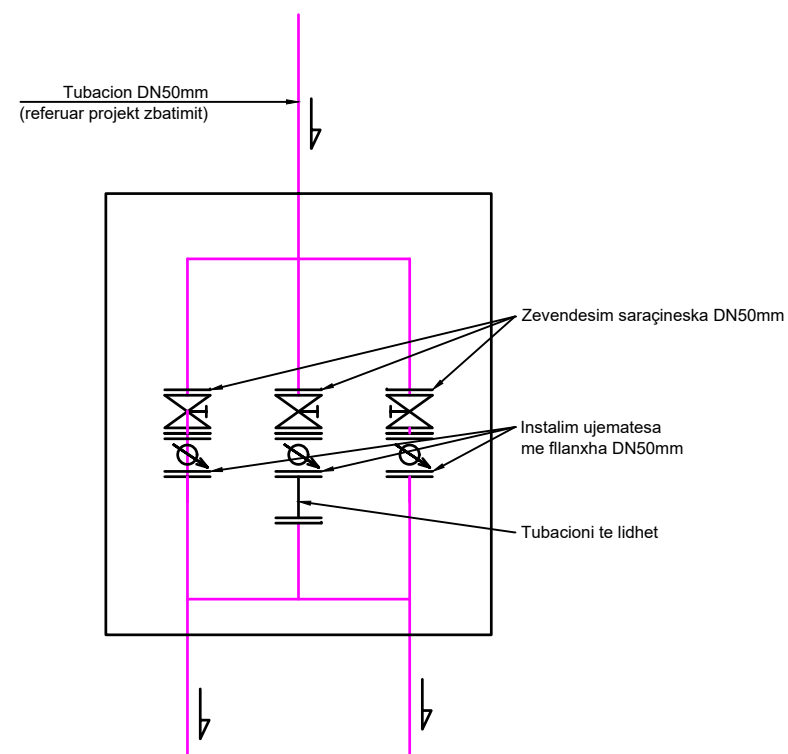
SKEMAT E PUSITES EKZISTUESE P2 (E PERFUNDUAR)
