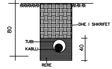
VENDOJA E KABLLIT TE FURNIZIMIT NEN TOKE
