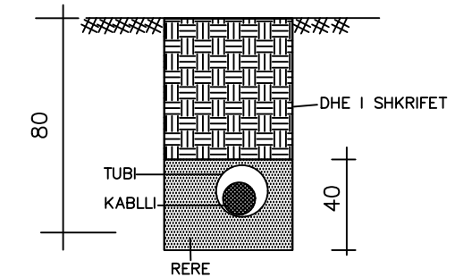
VENDOJA E KABLLIT TE FURNIZIMIT NEN TOKE
