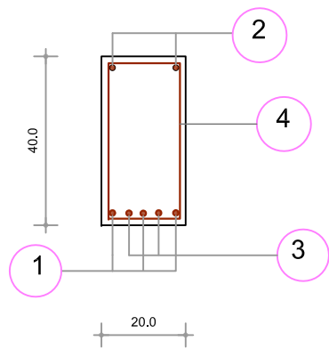
Prerja 1-1
