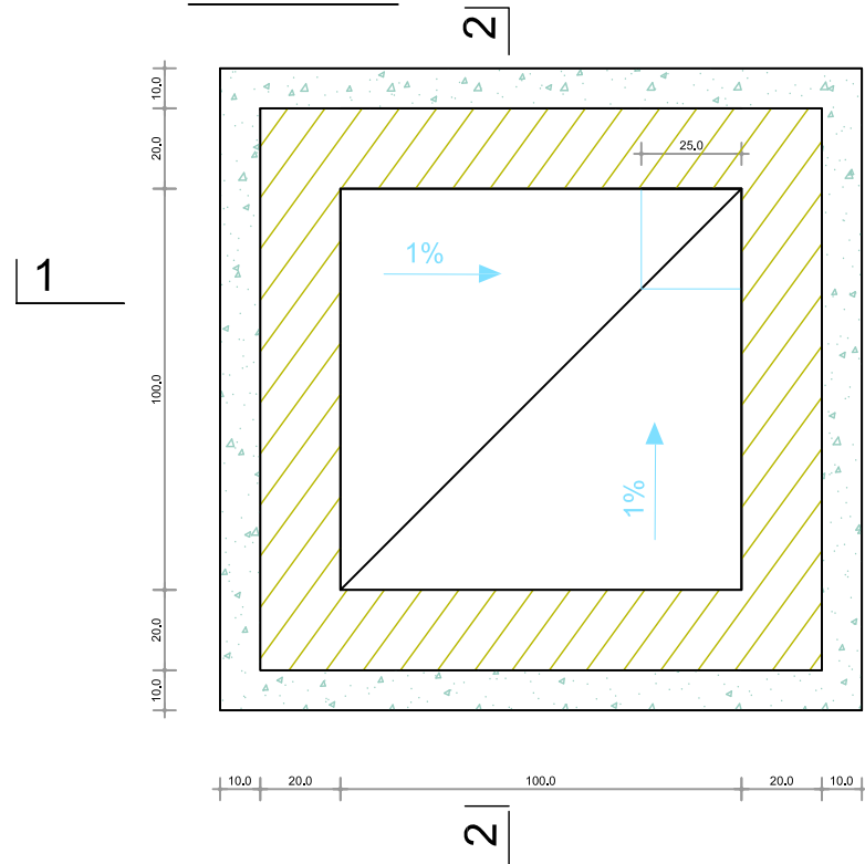
Planimetria shk 1:20
