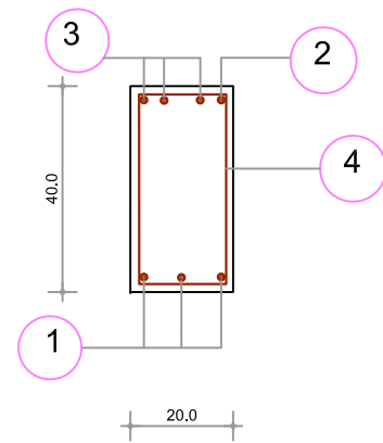
Prerja 2-2
