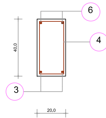
Prerja 3-3
