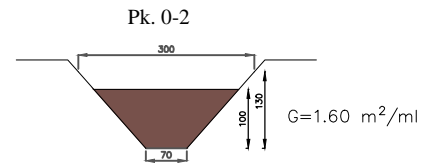
SEKSIONI TIP I VESHJES SE SHKARKUESIT Pk.0 +2, L=35 SH 1:50
