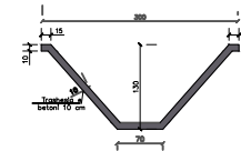
SEKSIONI TIP I VESHJES SE SHKARKUESIT Pk.0 +2, L=35 SH 1:50
