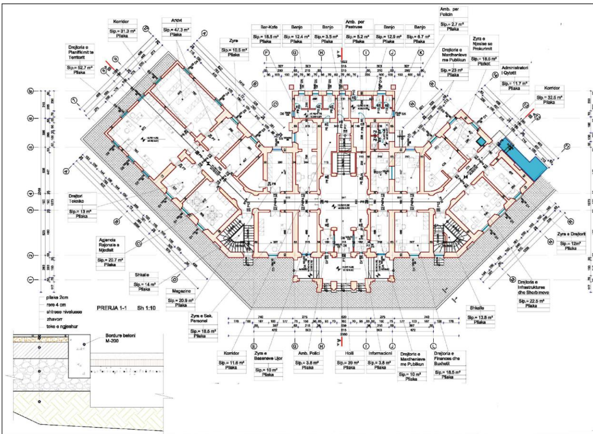
Planimetria e katit përdhe të objektit e marrë nga projekti i restaurimit i realizuar në 2017.
