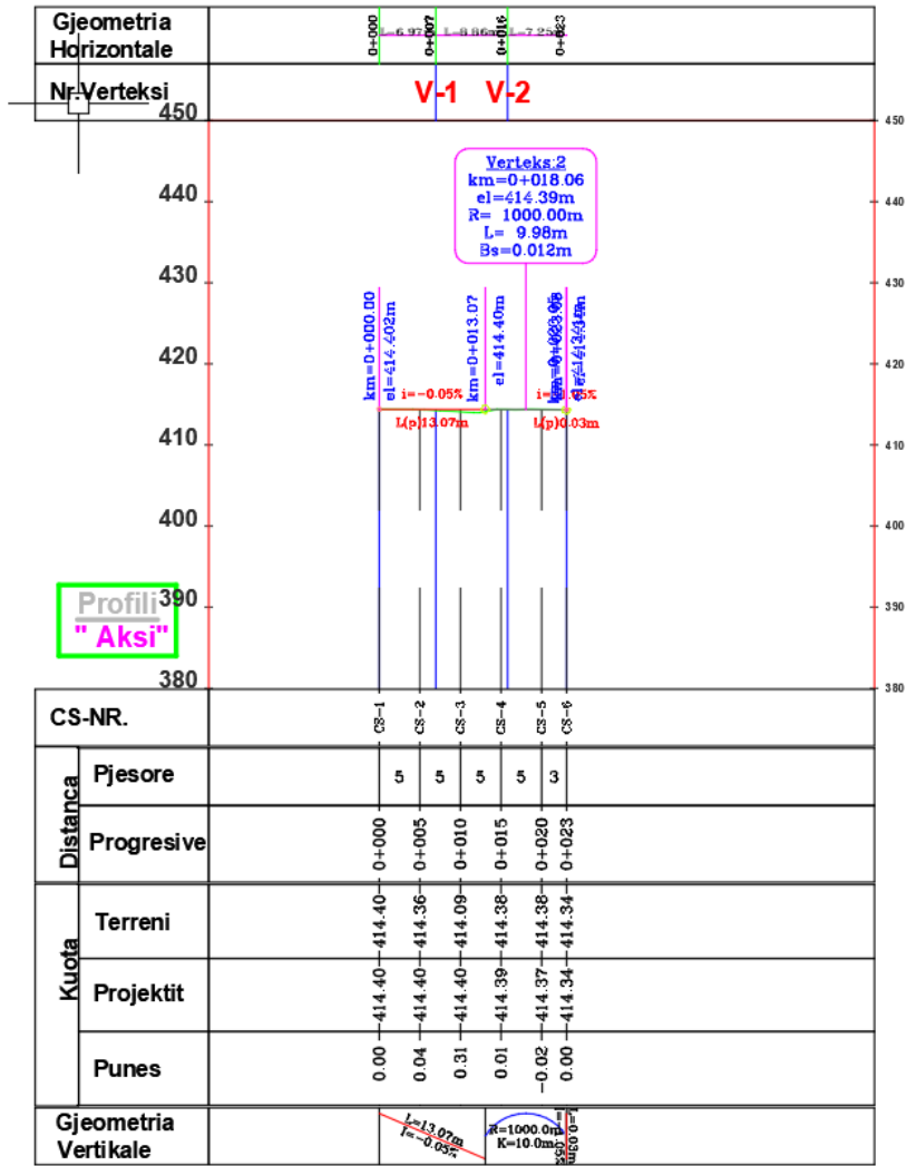
Figura 8: Profili gjatesor
