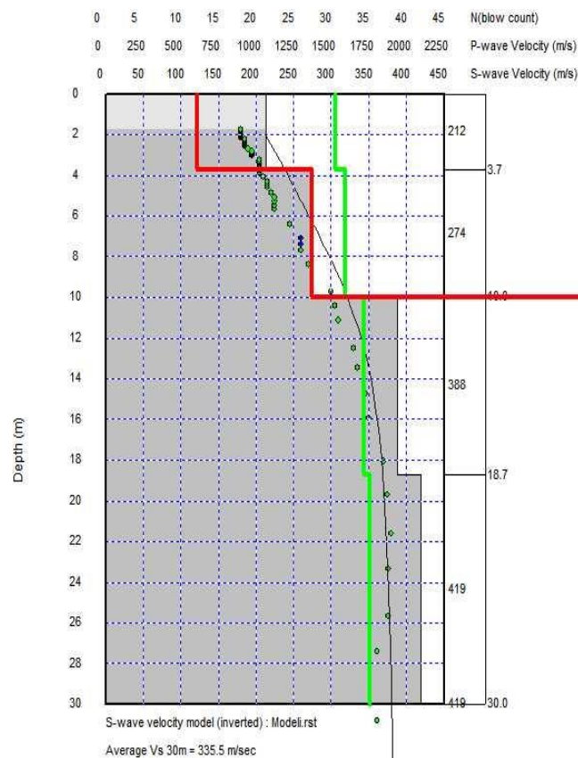
Figura 3. Kurba e ndryshimit të Vs në sheshin e ndërtimit dhe vlera e parametrit V_{s30}
