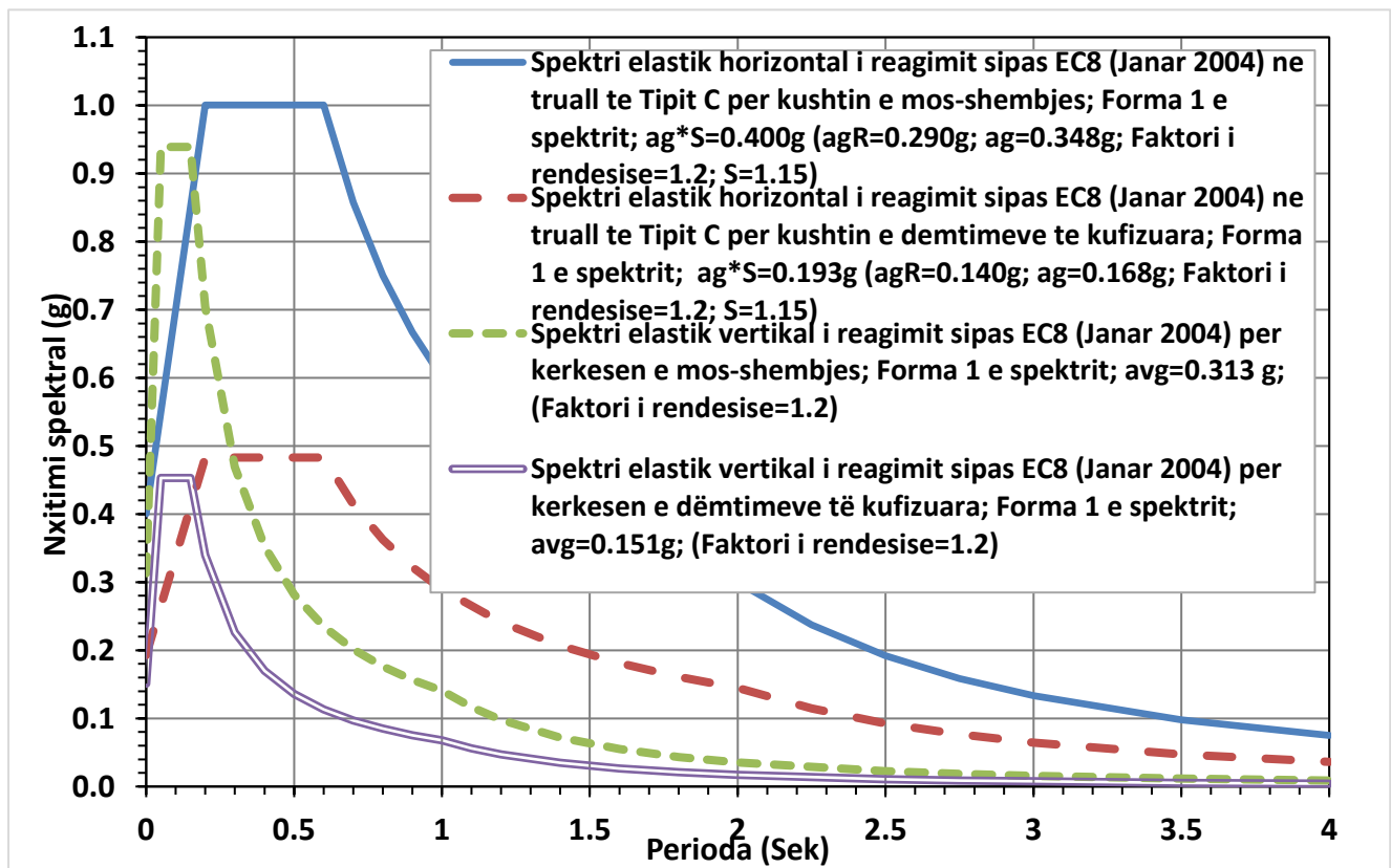
Figura 4. Spektrat elastikë horizontalë dhe vertikalë të reagimit për të dy nivelet e performancës sipas EC8 për objektin: Ndërtim Kopësht Çerdhe e integruar, në rrugën "Muharrem Caushi", Njësia Strukturore KA/208, Njësia Administrative Kashar, Bashkia Tiranë
