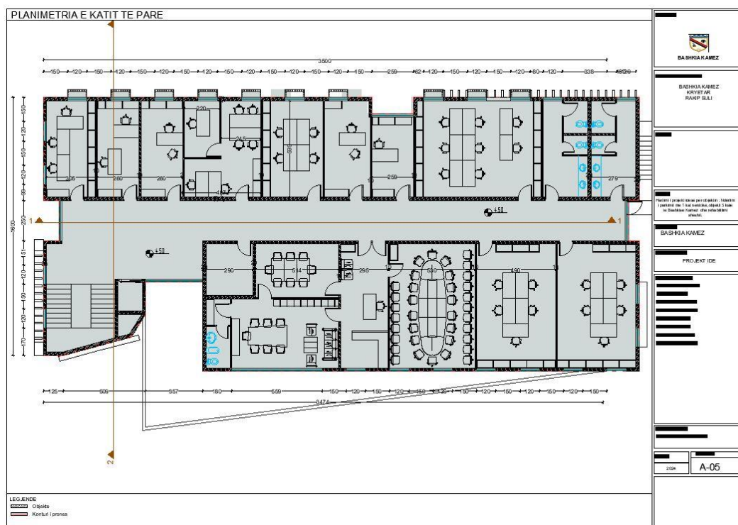
Plani i katit te pare
