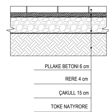
DETAJ 5 SH 1/20 SHIRMI I TROTUARAVE
