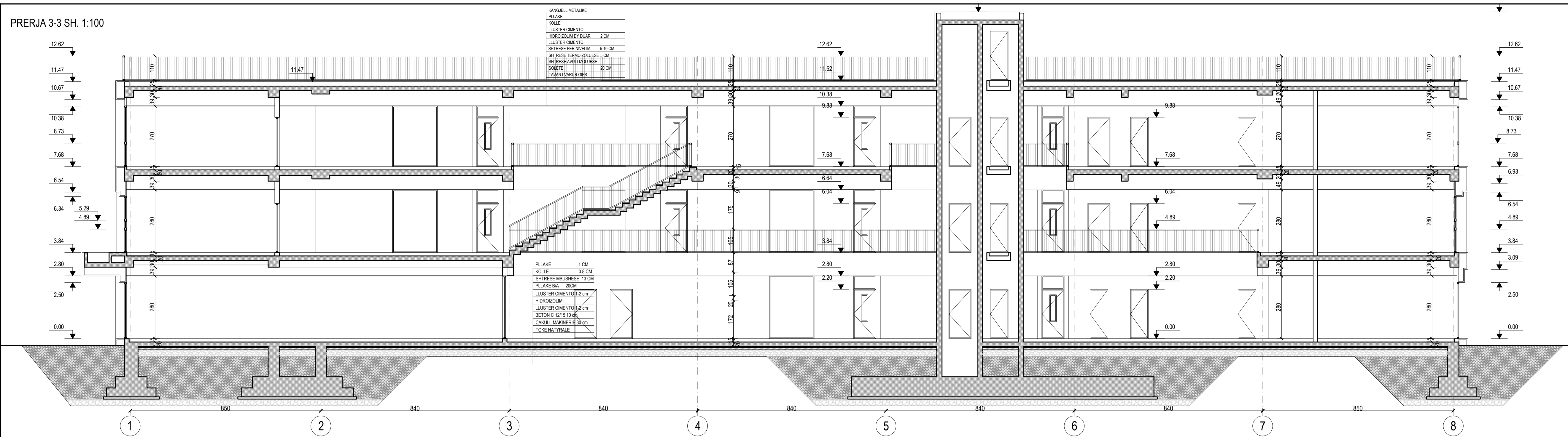
PRERJA A-A SH. 1:100
