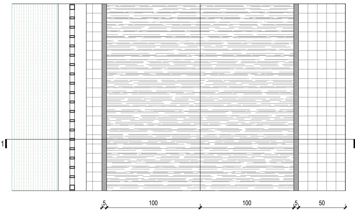
DETAJ 2 PISTA E VRAPIMIT SHK 1/25
