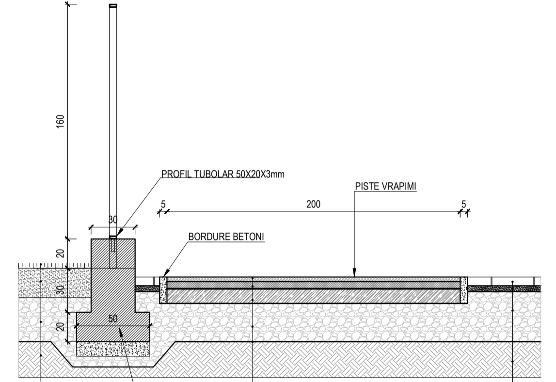
DETAJ 3 SH 1/25
