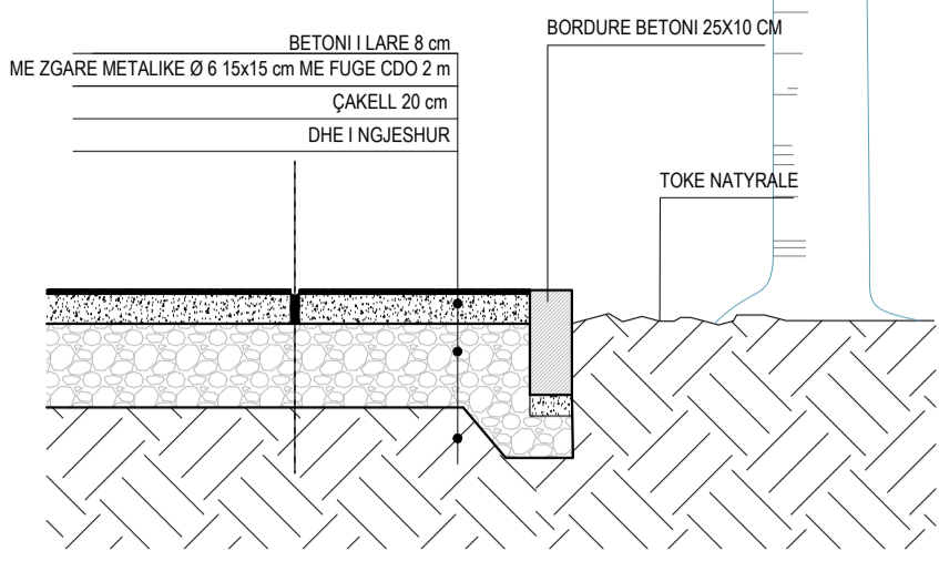
DETAJ 4 SH 1/20 SHIRMI I SHKREJTI
