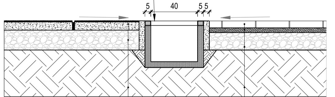
DETAJ 8 KOSH MBETURINASH SH 1/20
