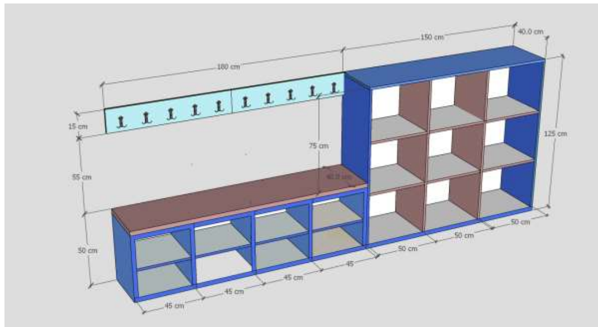
Fig.3. Modeli i raftit të pranimit (Fotot janë thjeshtë ilustruese, marka nuk është përcaktues definitiv, mund të ofertohet dhe ekuivalent i saj)
