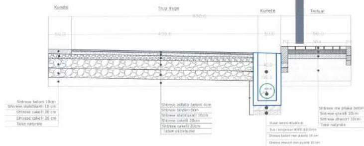
Prerja terthore e rruges me kunete
