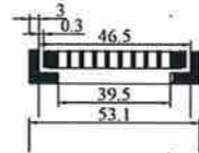
PRERJE B-B
