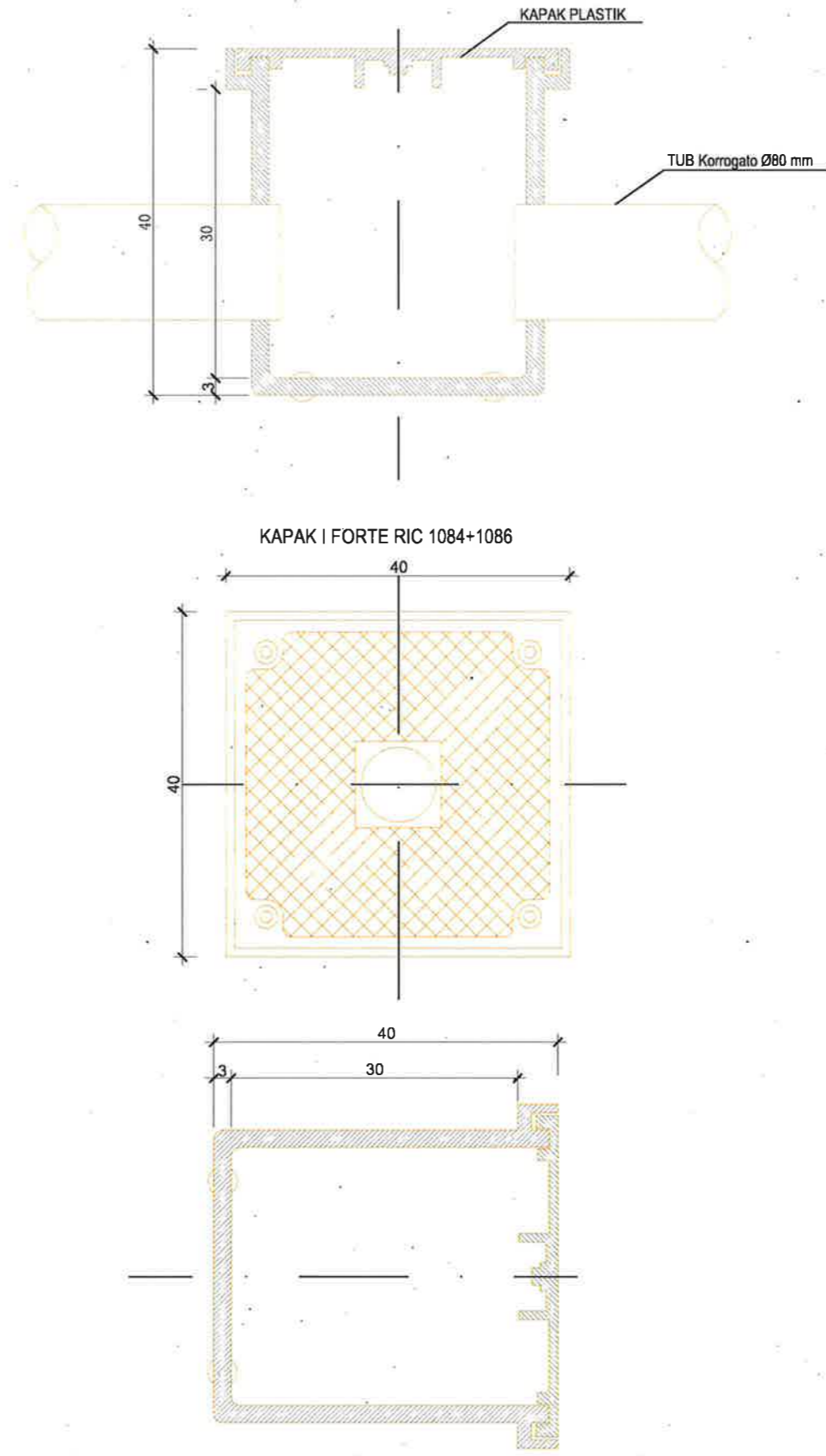
PLANI I DETAJIT TE PUSETES ,PLASTIKE 40X40X40 CM, SE NDRICIMIT DHE I MONTIMIT TE SAJ NE TOKE ME TUB
