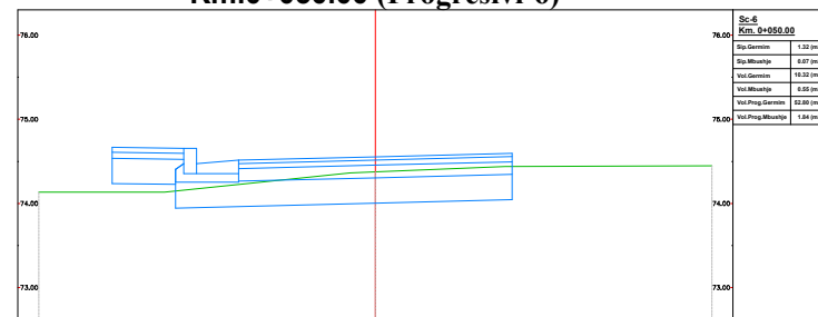
Km.0+050.00 (Progresivi-6)
