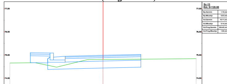
Km.0+120.00 (Progresivi-13)
