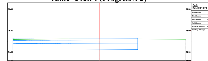
Km.0+018.71 (Progresivi-3)
