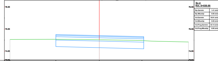
Km.0+030.00 (Progresivi-4)
