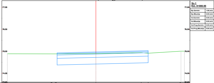
Km.0+000.00 (Progresivi-1)
