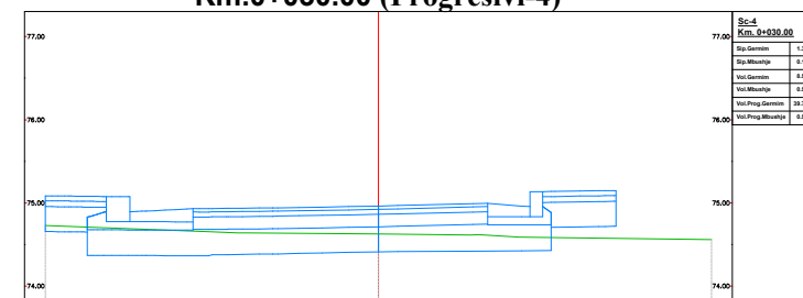
Km.0+030.00 (Progresivi-4)
