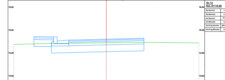
Km.0+110.00 (Progresivi-12)
