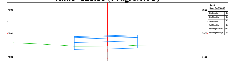
Km.0+020.00 (Progresivi-3)
