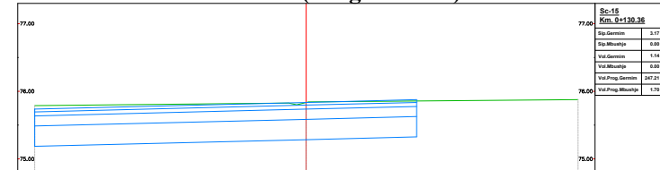
Km.0+130.36 (Progresivi-15)
