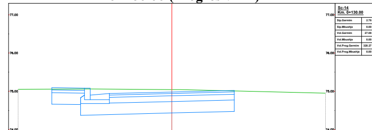
Km.0+130.00 (Progresivi-14)
