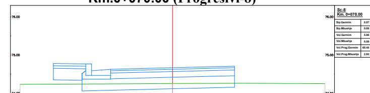
Km.0+070.00 (Progresivi-8)
