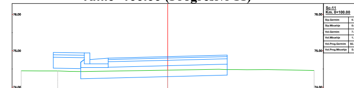
Km.0+100.00 (Progresivi-11)
