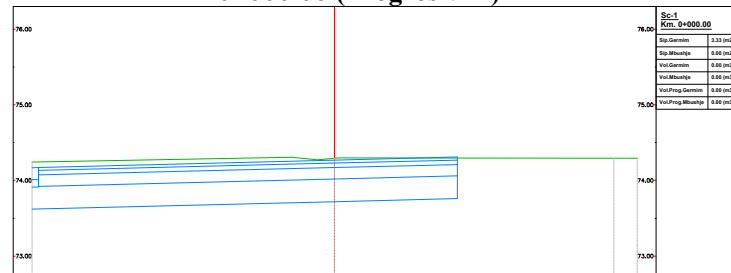
Km.0+000.00 (Progresivi-1)
