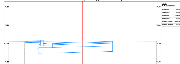
Km.0+080.00 (Progresivi-9)
