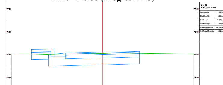
Km.0+120.00 (Progresivi-13)
