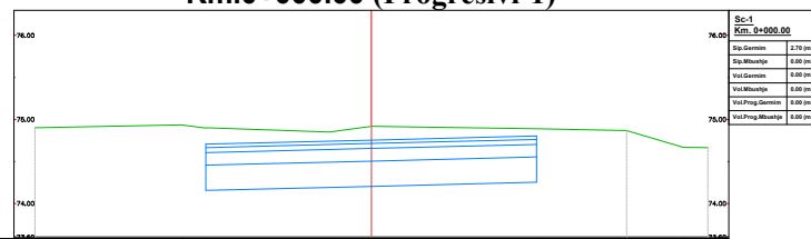
Km.0+000.00 (Progresivi-1)
