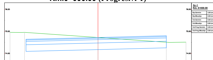
Km.0+000.00 (Progresivi-1)
