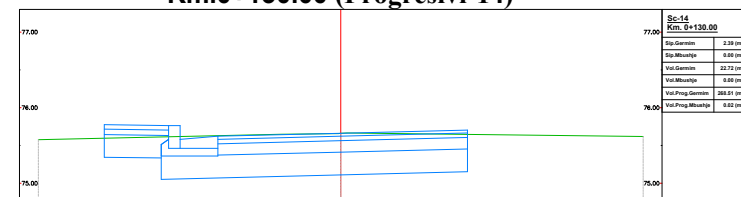
Km.0+130.00 (Progresivi-14)
