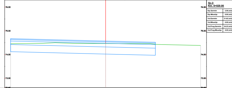
Km.0+020.00 (Progresivi-3)
