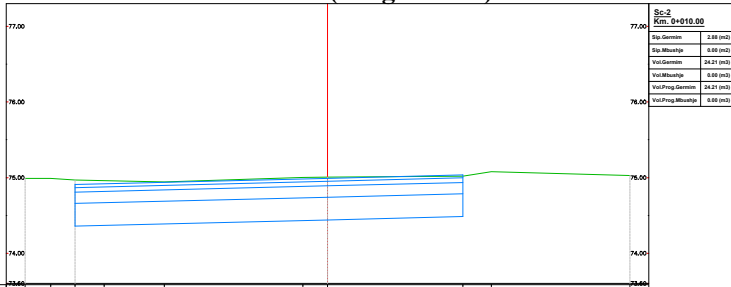
Km.0+010.00 (Progresivi-2)
