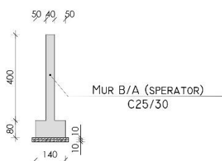
PRERJA 1 - 1 E SPERATORËVE SHK. 1 : 100
