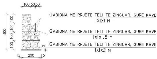
PRERJA 2 - 2 E MURE SHK. 1 : 100
