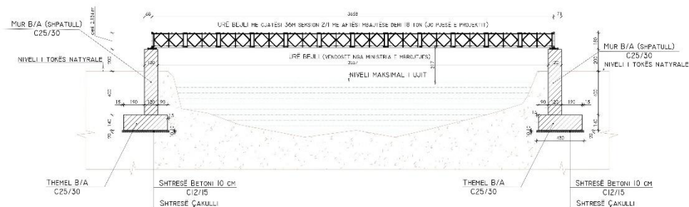
PRERJA SIPAS AKSIT TË URËS SHK. 1 : 200
