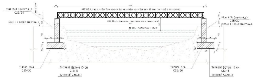
PRERJA SIPAS AKSIT TË URËS SHK. 1 : 200
