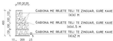
PRERJA 2 - 2 E MURE SHK. 1 : 100
