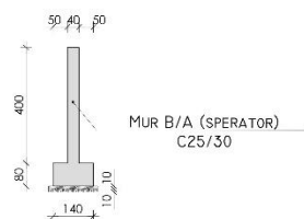
PRERJA 1 - 1 E SPERATORËVE SHK. 1 : 100
