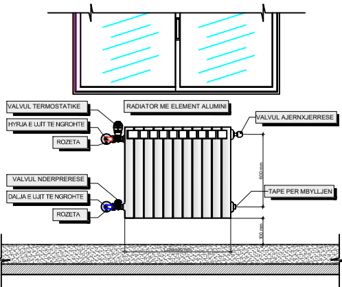
DETALJ I MONTIMIT TË RADIATORIT
