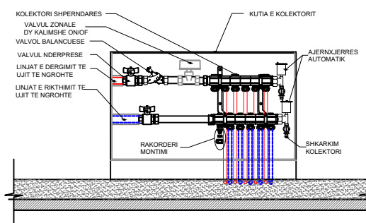
DETALJ I KUTISË SE KOLEKTORIT SHPËRNDARËS
