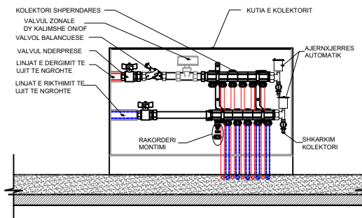
DETALJ I KUTIESE SE KOLEKTOREVE SHPERNDARES
