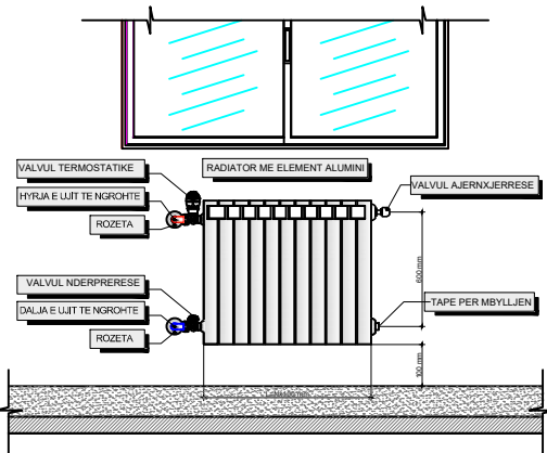
DETALJ MONTIMI I RADIATORIT
