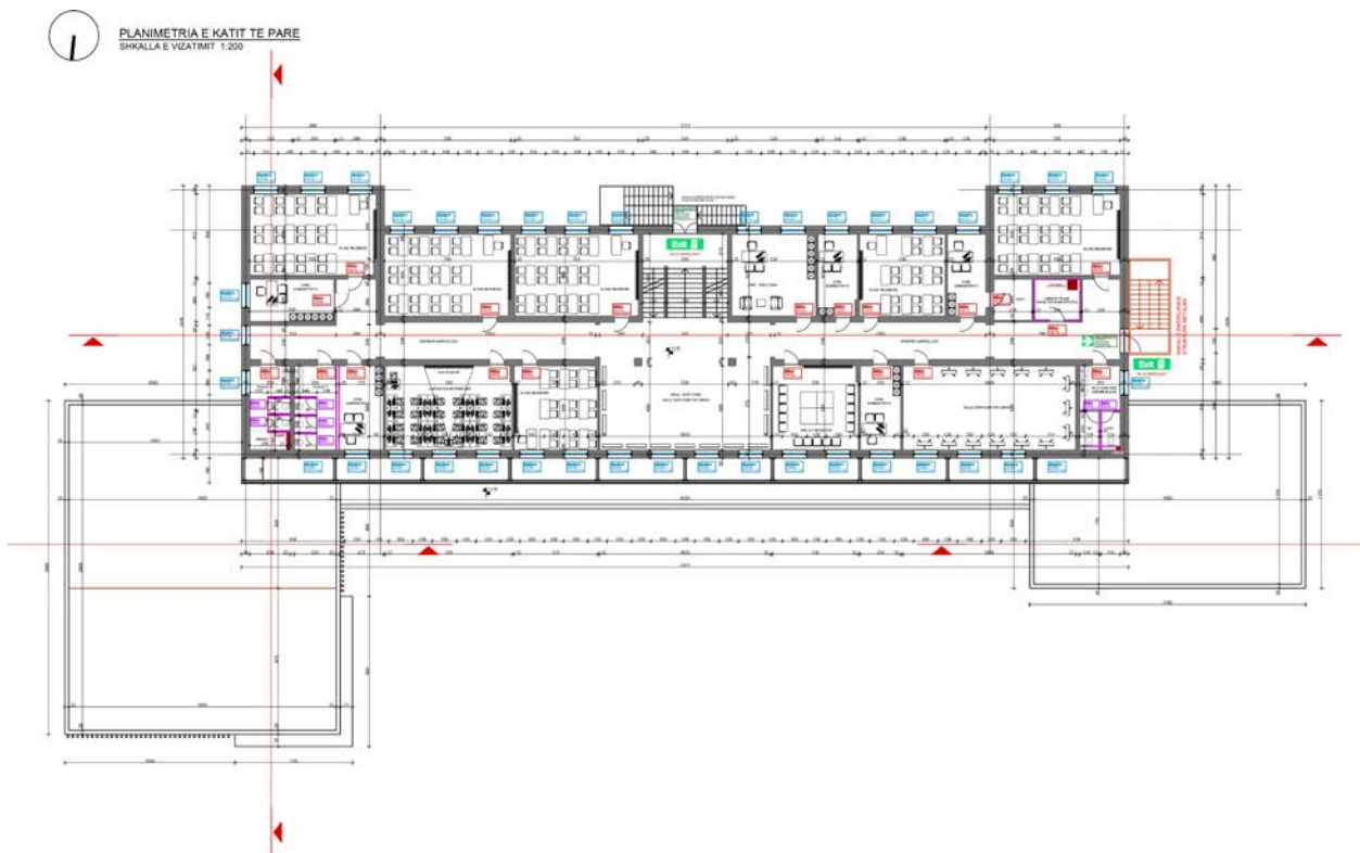
Fig.6 – Planimetria e Katit te Pare / Plani I Propozuar
