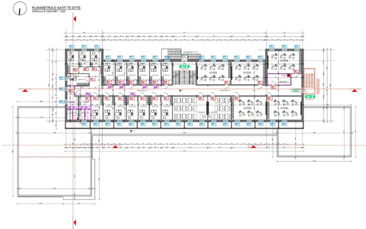
Fig.7 – Planimetria e Katit te Dyte / Plani I Propozuar
