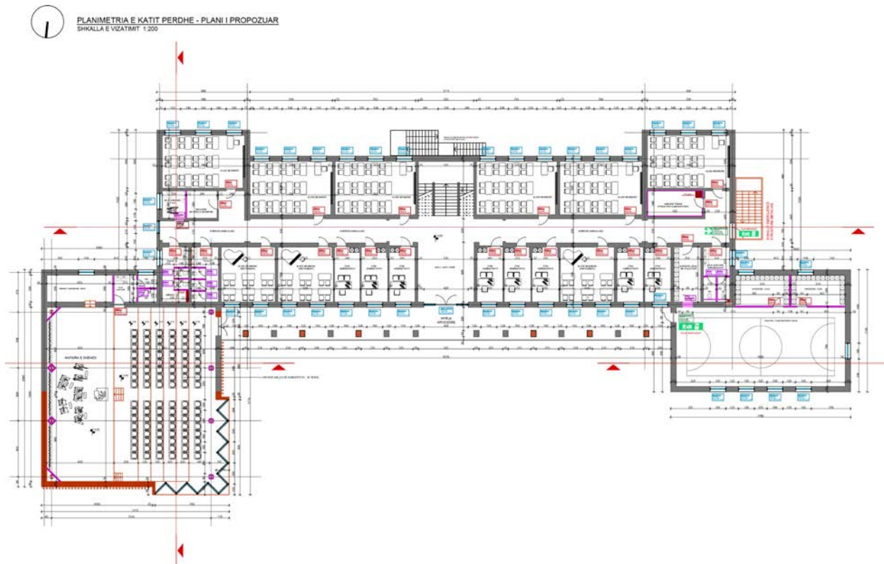
Fig.5 – Planimetria e Katit Perdhe / Plani I Propozuar
