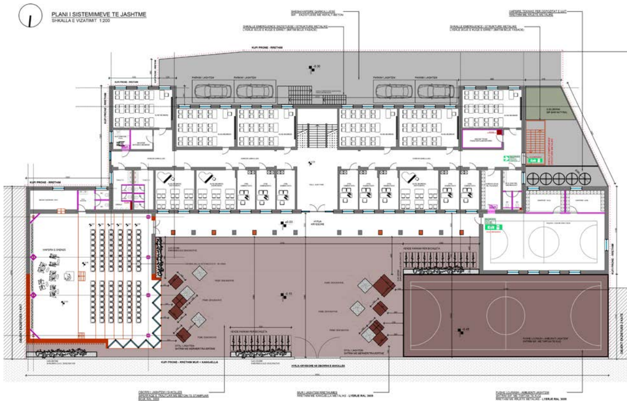
Fig.8 – Planimetria e Sistemeve te Jashtme / Plani I Propozuar
