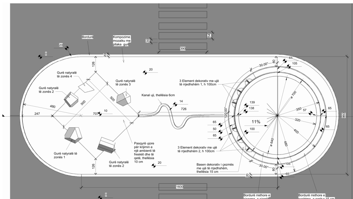
Figura 4. Plansistemimi i përgjithshëm me elementet kryesore: gurë natyralë, pasqyrë ujore, kanal uji, bordura dhe burim.
