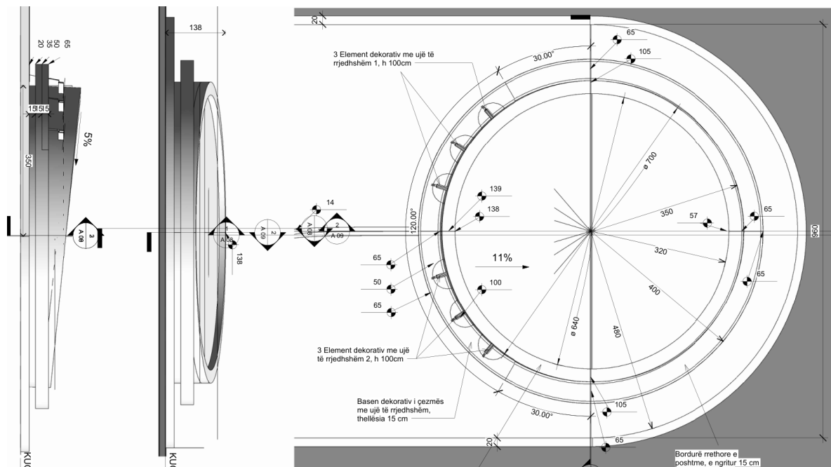
Figura 6. Plan dhe prerje e strukturës së burimit dhe elementeve me ujë.
