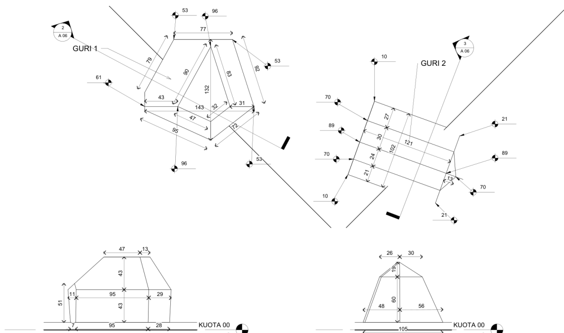
Figura 5. Detaje dhe prerje të gurëve natyralë dekorativë.
