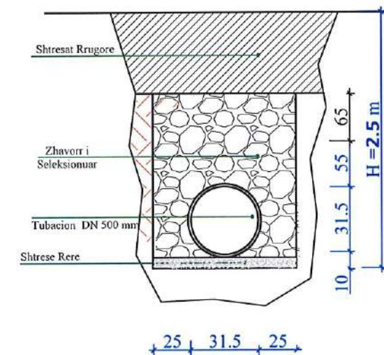
PRERJE TERTHORE KANALI Tubacion DN 500 mm (H = 2.5m) SH 1:20
