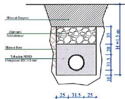
PRERJE TERTHORE KANALI Tubacion PEHD i brinjezuar DN 315 mm (H deri 1.5m) SH 1:20
