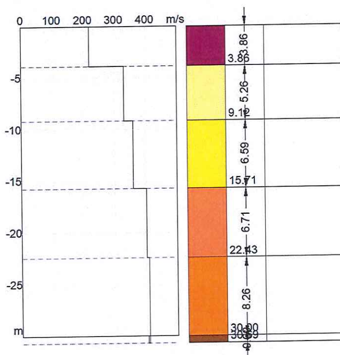
Figura 13. Profili i shpërndarjes së valëve ( V_s ) me thellësinë dhe përfitim i modelit gjeologo-inxhinierik të sheshit të ndërtimit
