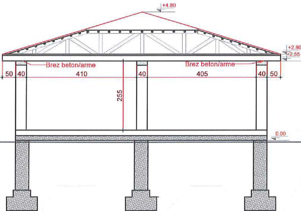
Fasada e Objektit
