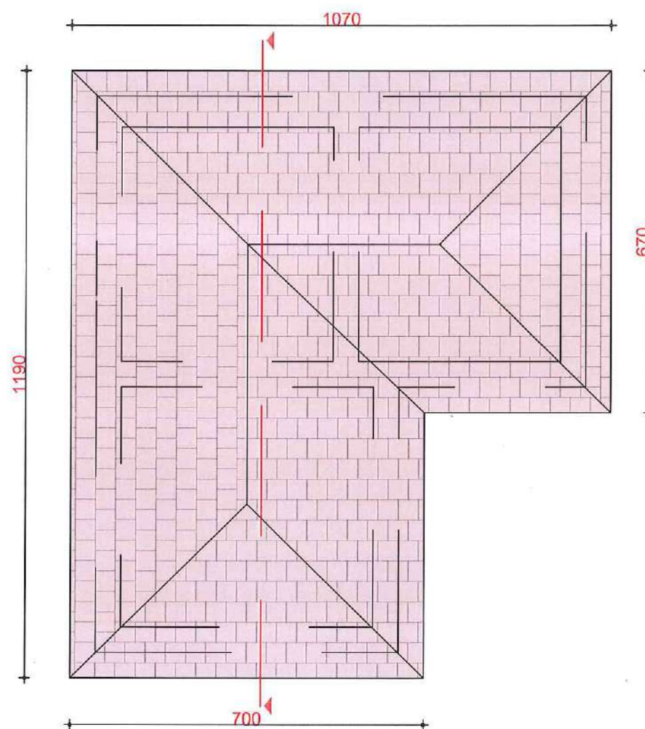
Planimetria e Çatisë
