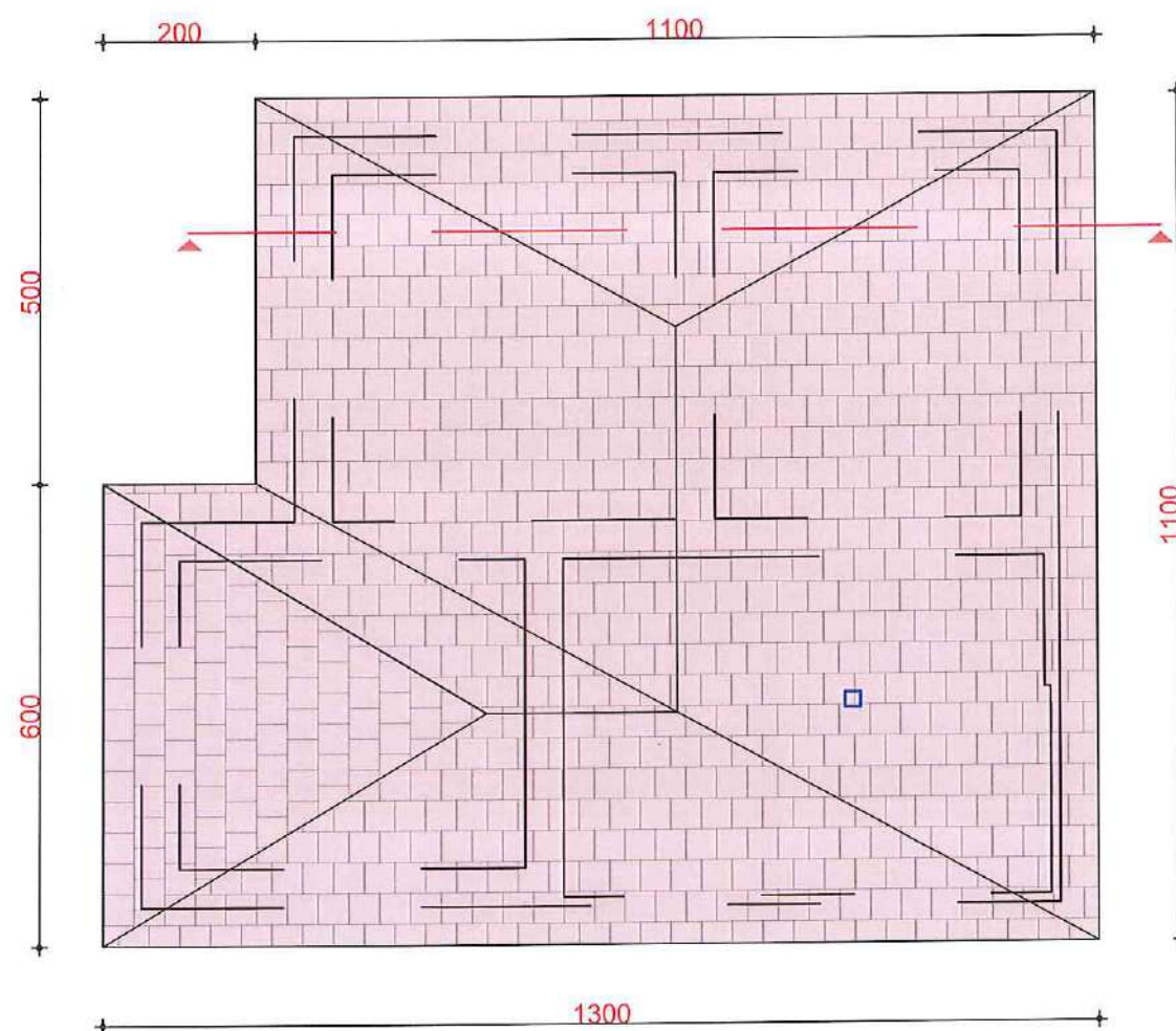
Planimetria e Çatisë
