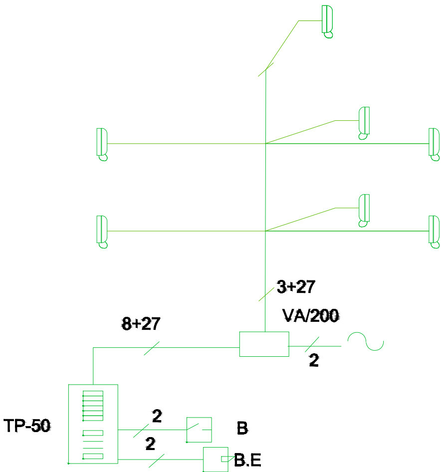
SKEMA E CITOFONISE
