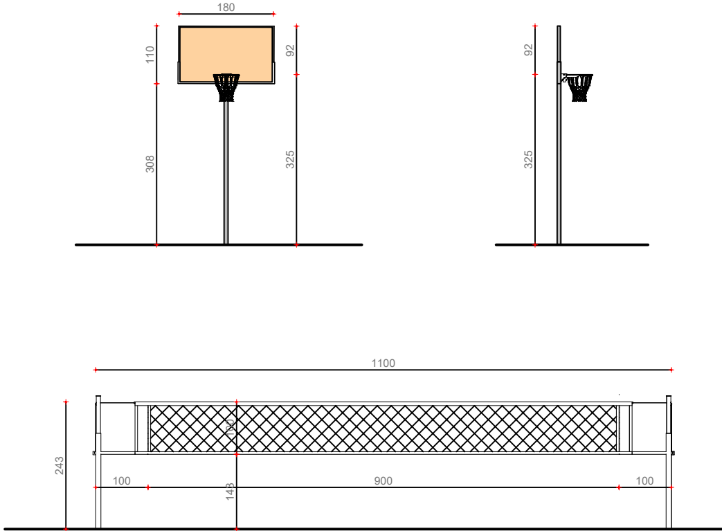
DETAJE TE KOSHIT TE BASKETBALLIT DHE RRJETES
