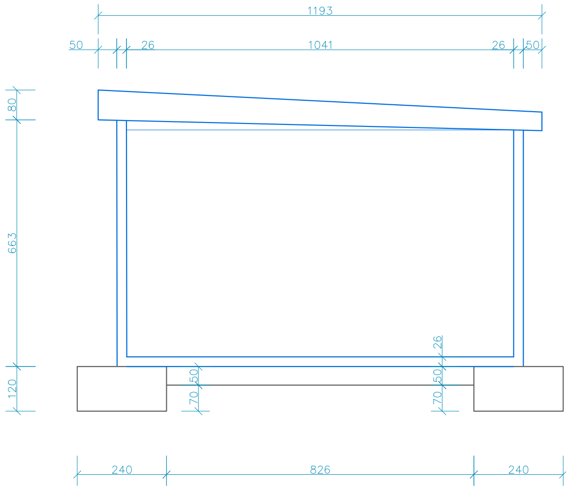
PALESTRA - KONSTRUKSIONI METALIK DHE PLINTAT B/A, SH-1:100
