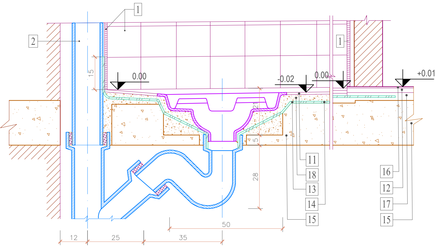
Prerja "c - c"
