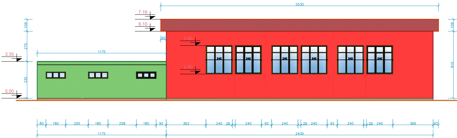
PAMJE E FSADES NGA VERIU
