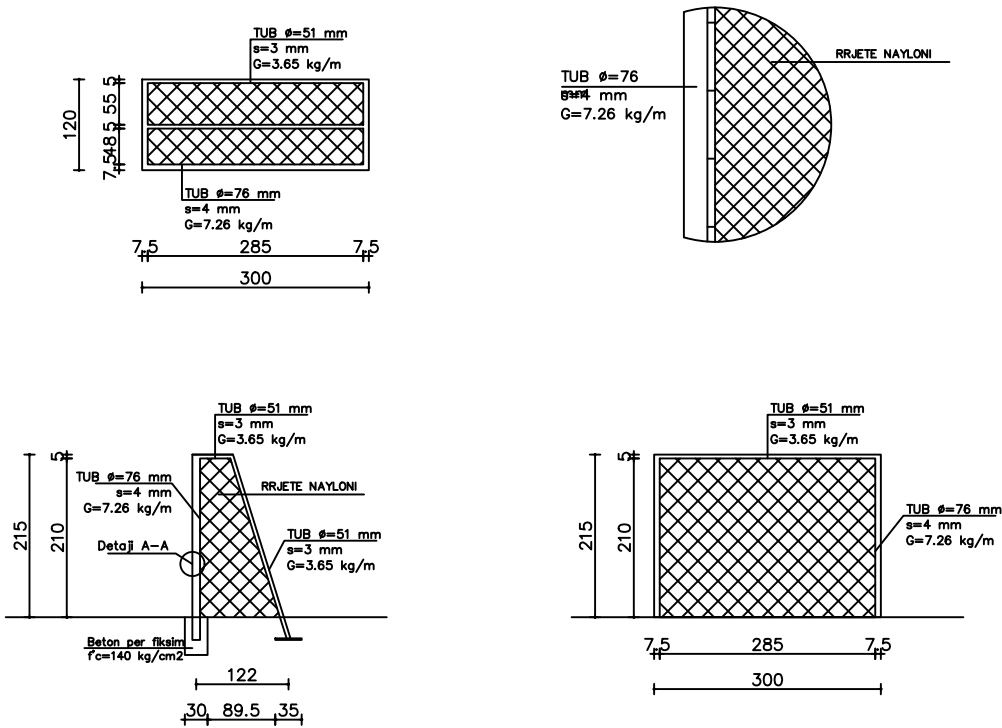
DETAJI I PORTSES SE FUTBOLLIT
